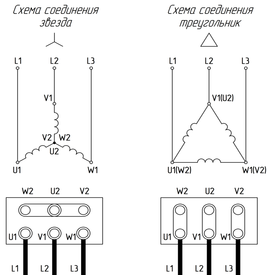
Рис. 2 Схемы подключения питания для трехфазного асинхронного двигателя
