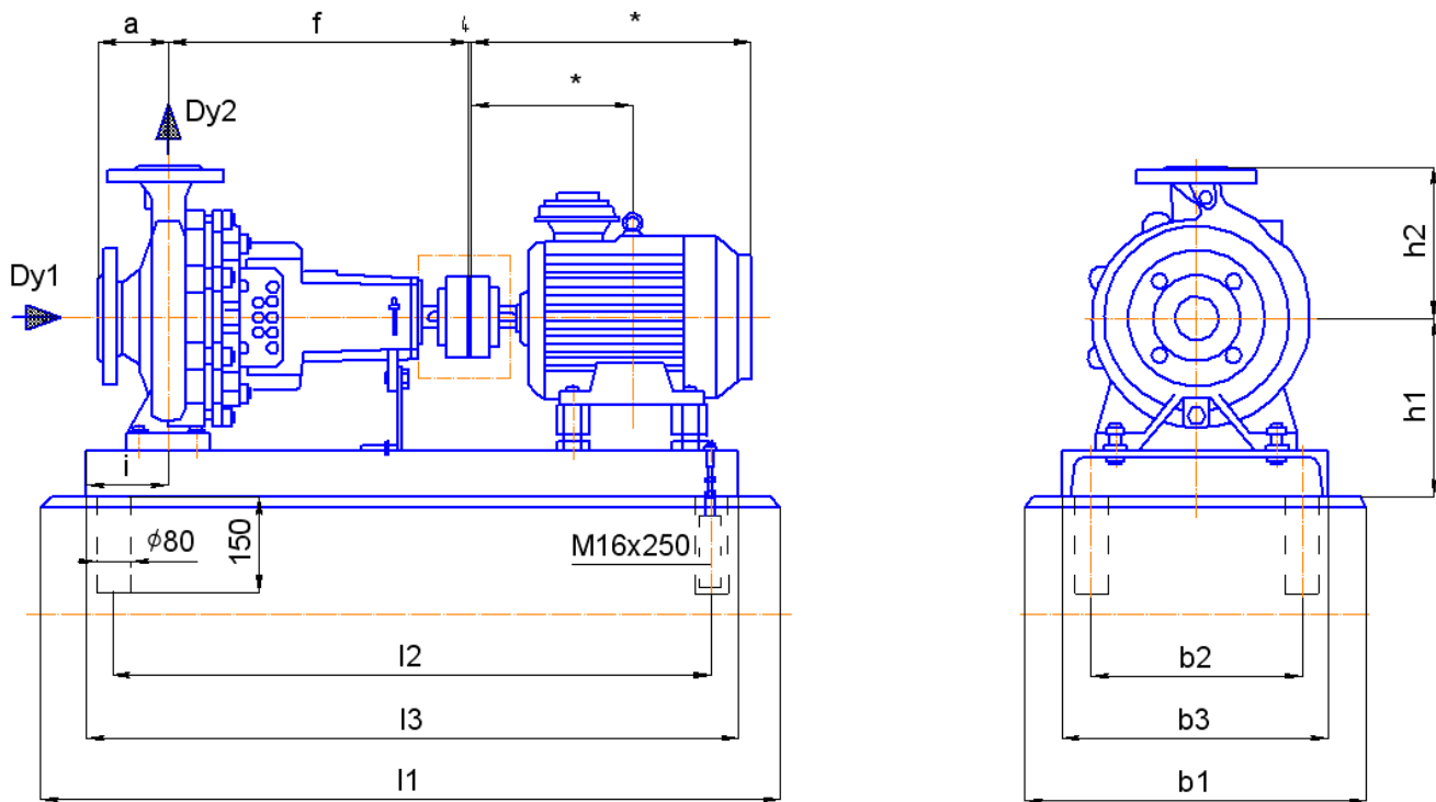
Рисунок 5. Габаритные и присоединительные размеры Иртыш – ЦНК - Ех.
