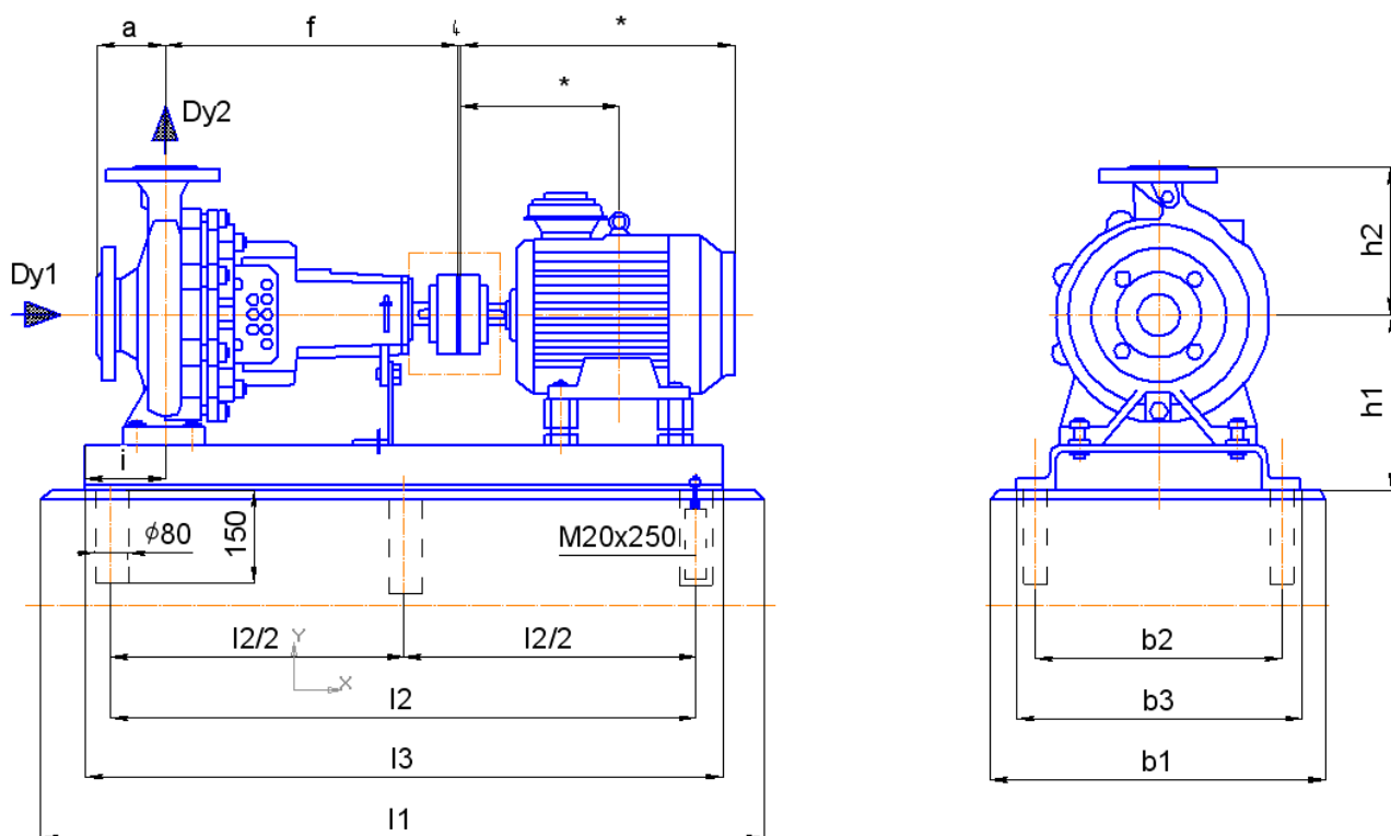
Рисунок 5. Габаритные и присоединительные размеры Иртыш – ЦНК - Ех.
