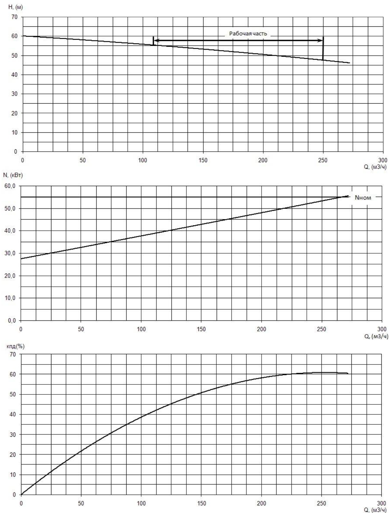
Рис. 1. Рабочие характеристики: для электронасоса Иртыш НФ2 125/400.406-55/4Ex-400
