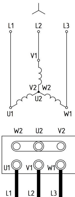
Рис. 4 Схемы подключения питания для трехфазного асинхронного двигателя
