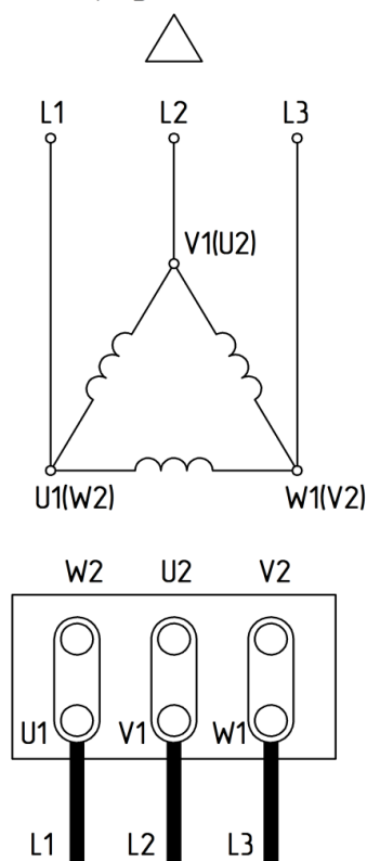
Рис. 4 Схемы подключения питания для трехфазного асинхронного двигателя
