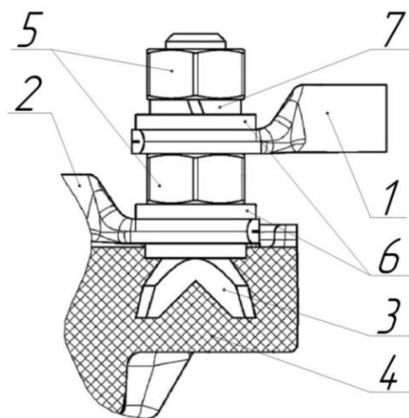
Рис. 3 Схема контактного соединения
