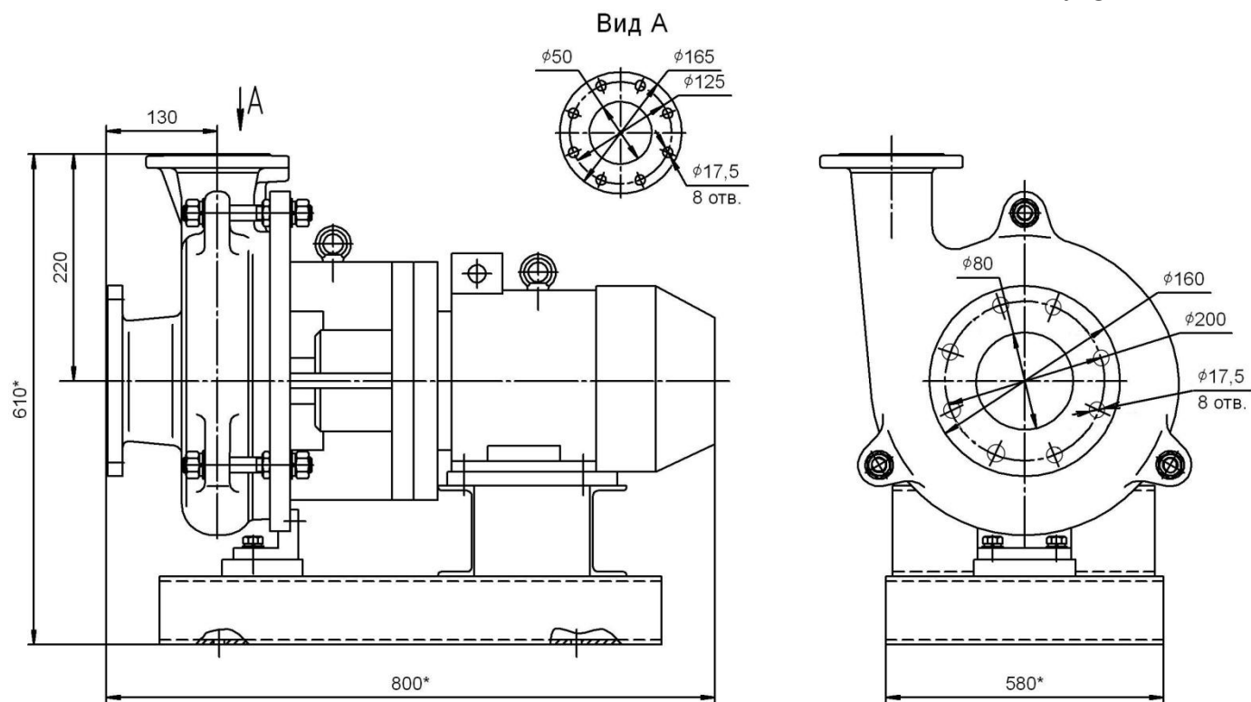
Рис. 4 Габаритные и присоединительные размеры электронасоса Иртыш НШ6 50/320.320-11/4Ех-200
