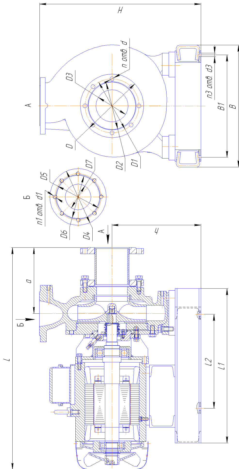
Рис. 7. Габаритные и присоединительные размеры электронасоса серии Иртыш НШ Ex– 200;
