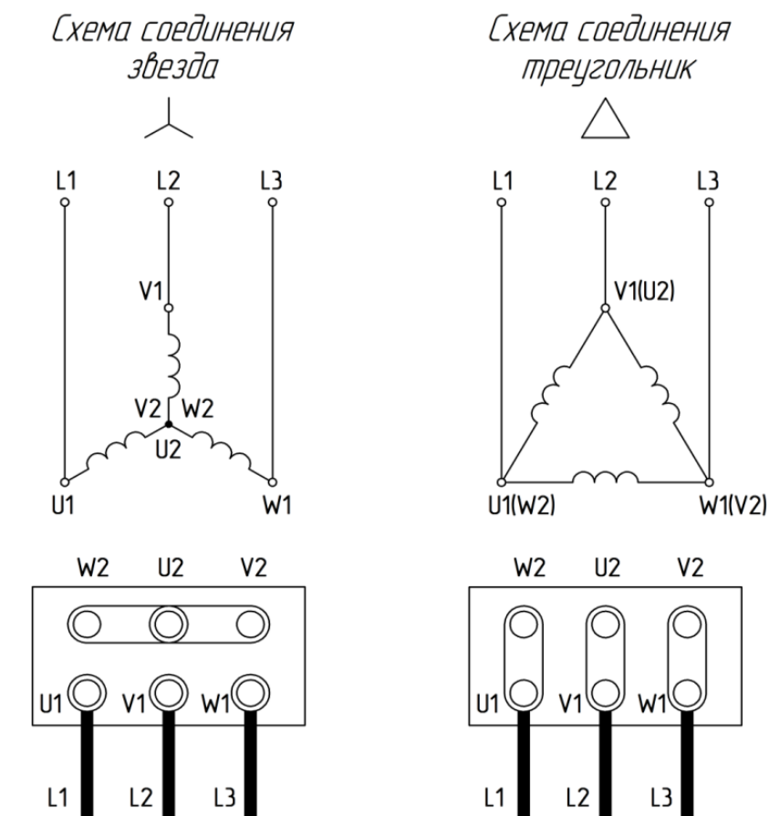
Рис. 3 Схемы подключения питания для трехфазного асинхронного двигателя
