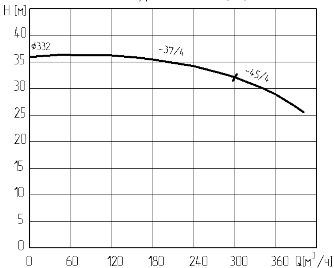
Рис. 9 Рабочие характеристики насоса «Иртыш»: ПД 150/315.332 – 37/4; ПД 150/315.332 – 45/4;
