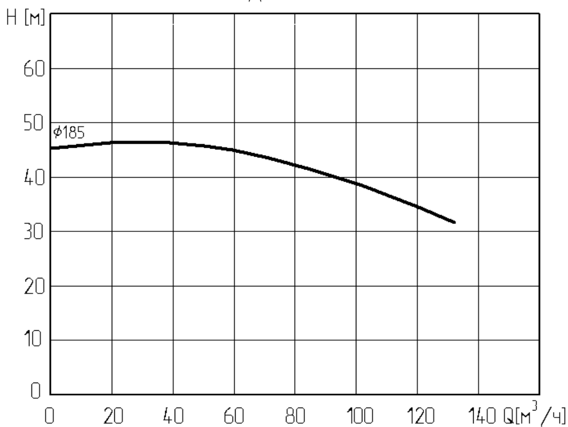
Рис. 3 Рабочие характеристики насоса «Иртыш»:
