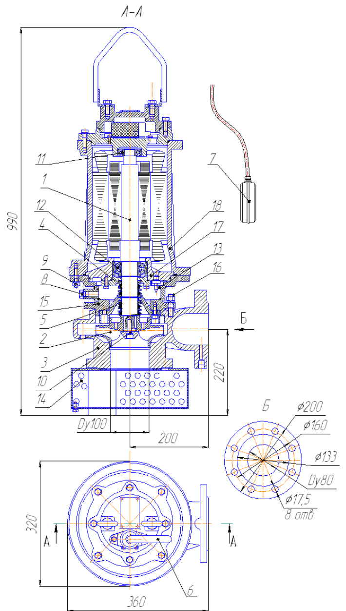
Рис. 22 Общий вид, габаритные и присоединительные размеры электронасоса "Иртыш" ПД 80/160 – 11/2
