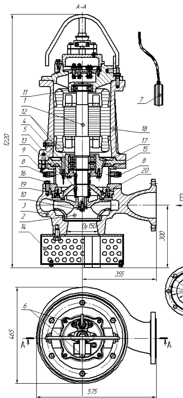
Рис. 25 Общий вид, габаритные и присоединительные размеры электронасоса «Иртыш» ПД 125/250 – 15/4
