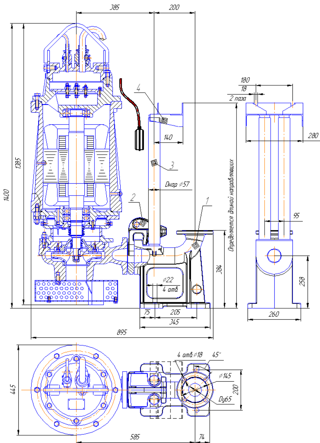
Рис. 39 Общий вид и габаритные размеры электронасоса "Иртыш" ПД 65/250 – 37/2 с опускным устройством.
