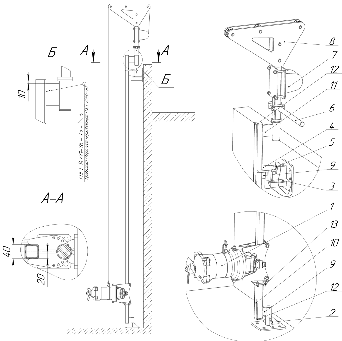
Рис. 4 Общий вид электромешалки "Иртыш" ПМЗ 188 – 0,75/4
