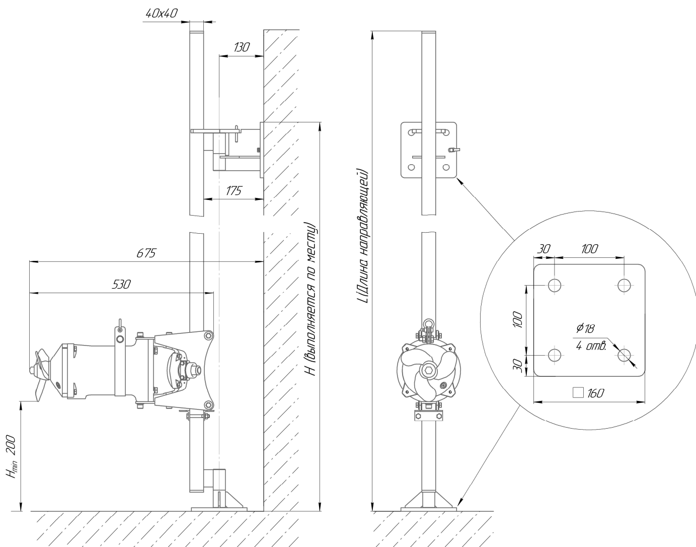
Рис. 5 Габаритные и монтажные размеры электромешалки "Иртыш" ПМЗ 188 – 0,75/4 с поворотным опускным устройством (без подъёмного устройства)
