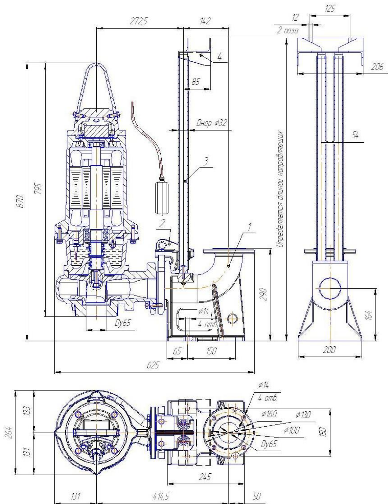
Рис. 80 Общий вид и габаритные размеры электронасоса "Иртыш" ПФ2 65/180 – 4/2– 106; ПФ2 65/180 – 5,5/2 – 106 с опускным устройством
