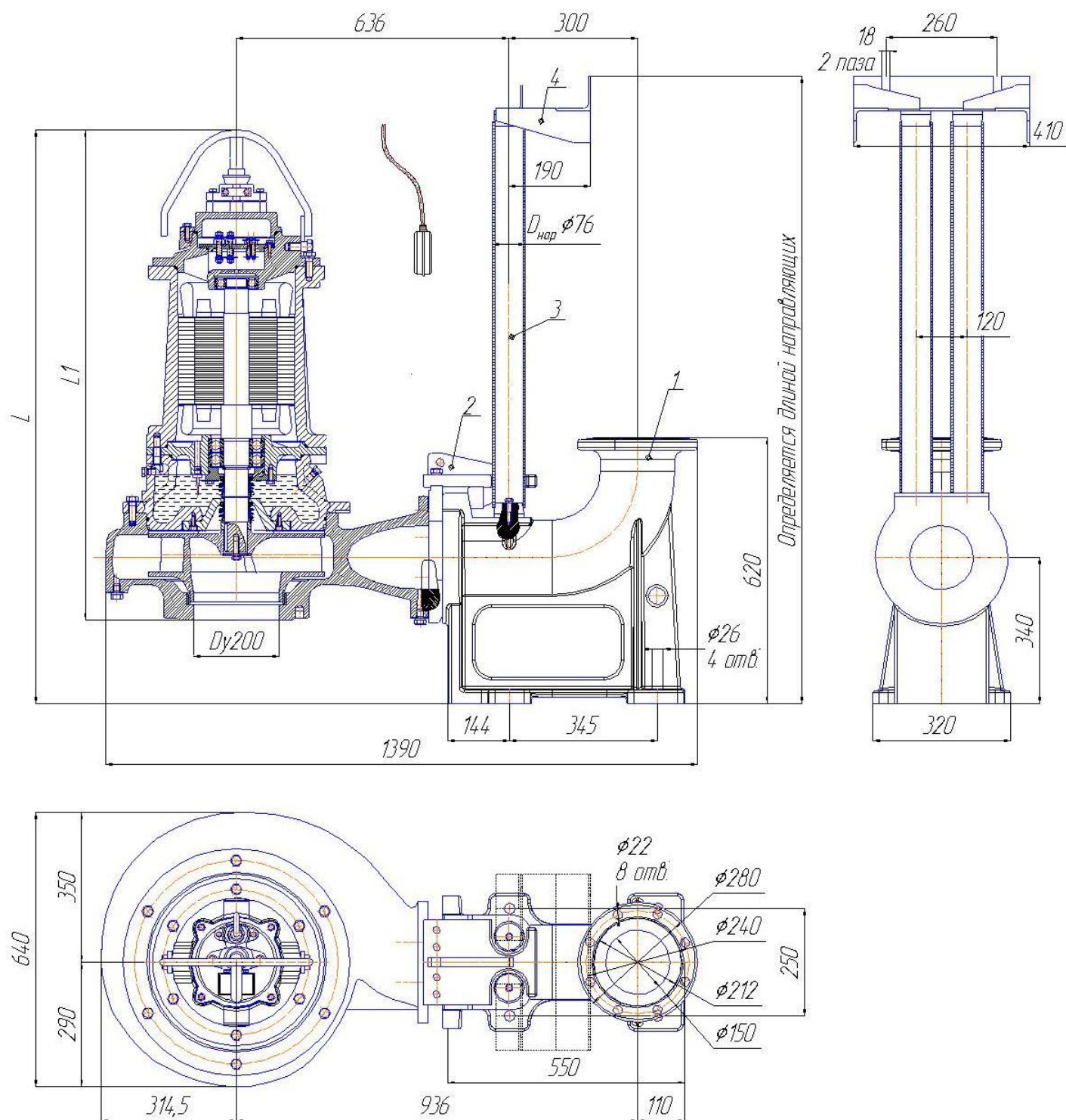
Рис. 105 Общий вид и габаритные размеры электронасоса "Иртыш" ПФЗ 150/400 – 15/6– 106; ПФЗ 150/400 – 18,5/6– 106 с опускающим устройством.
