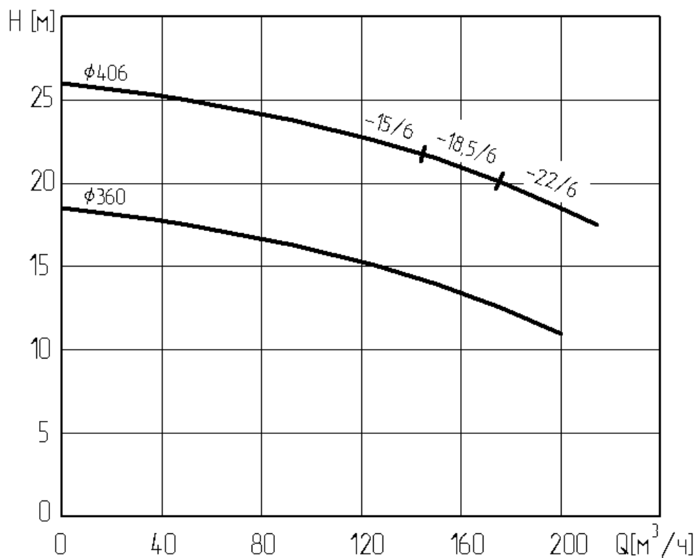
Рис. 11 Рабочие характеристики насоса «Иртыш»: ПФ2 125/400.360 – 11/ 6, ПФ2 125/400.406 – 15/ 6 ПФ2 125/400.406 – 18,5/6, ПФ2 125/400.406 – 22/ 6
