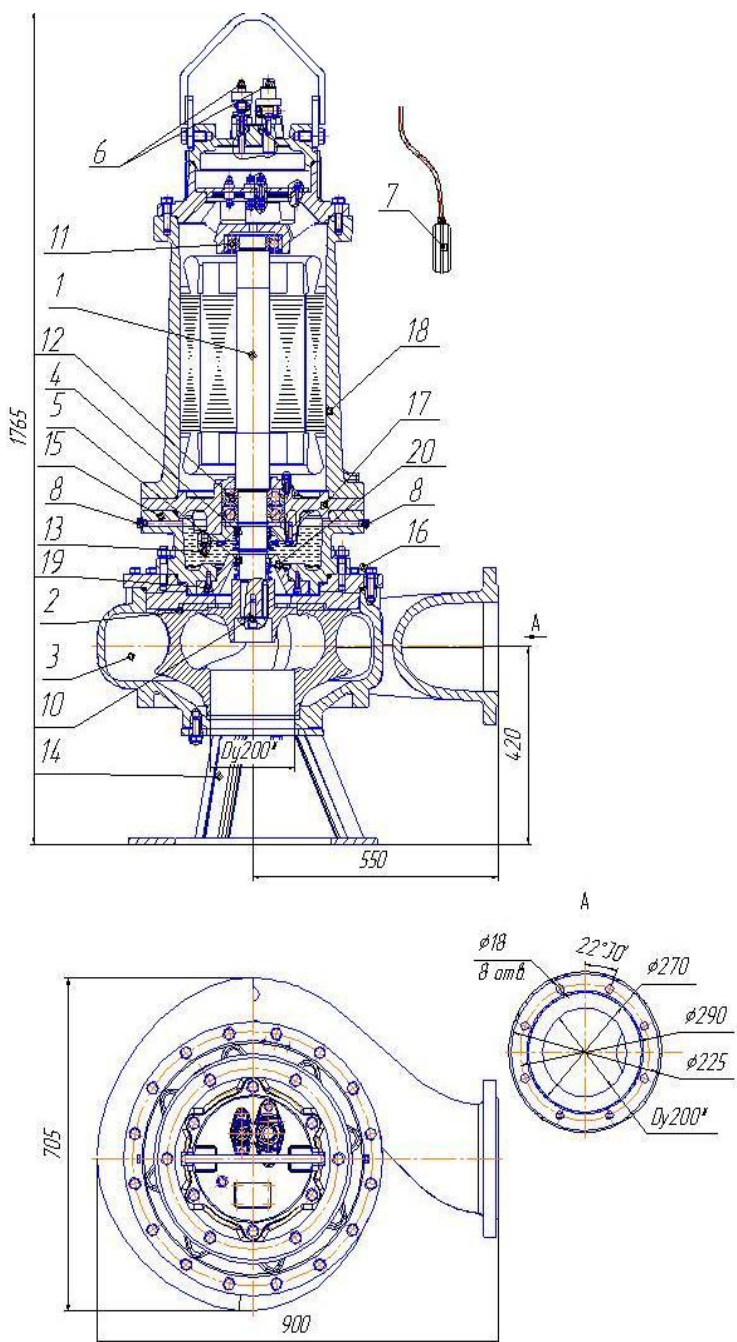
Рис. 62 Общий вид, габаритные и присоединительные размеры электронасоса "Иртыш" ПФ2 200/450 – 37/6;
