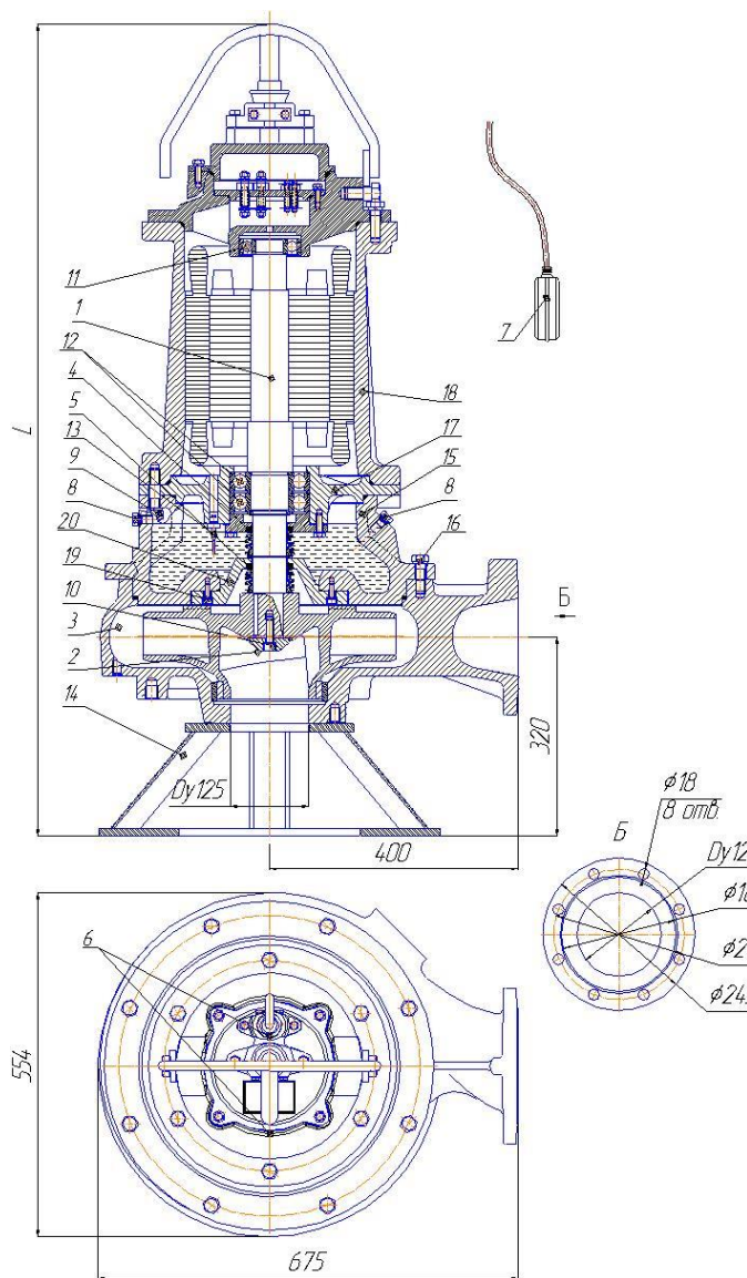
Рис. 49 Общий вид, габаритные и присоединительные размеры электронасоса "Иртыш" ПФ2 125/400 – 11/6; ПФ2 125/400 – 15/6; ПФ2 125/400 – 18,5/6.
