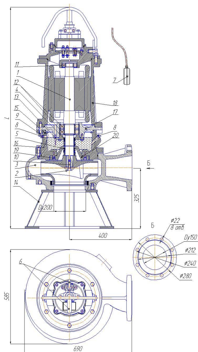
Рис. 54 Общий вид, габаритные и присоединительные размеры электронасоса "Иртыш" ПФ2 150/315–11/6; ПФ2 150/315–15/6; ПФ2 150/315–18,5/6.
