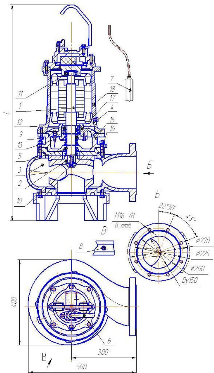
Рис. 51 Общий вид, габаритные и присоединительные размеры электронасоса "Иртыш"
