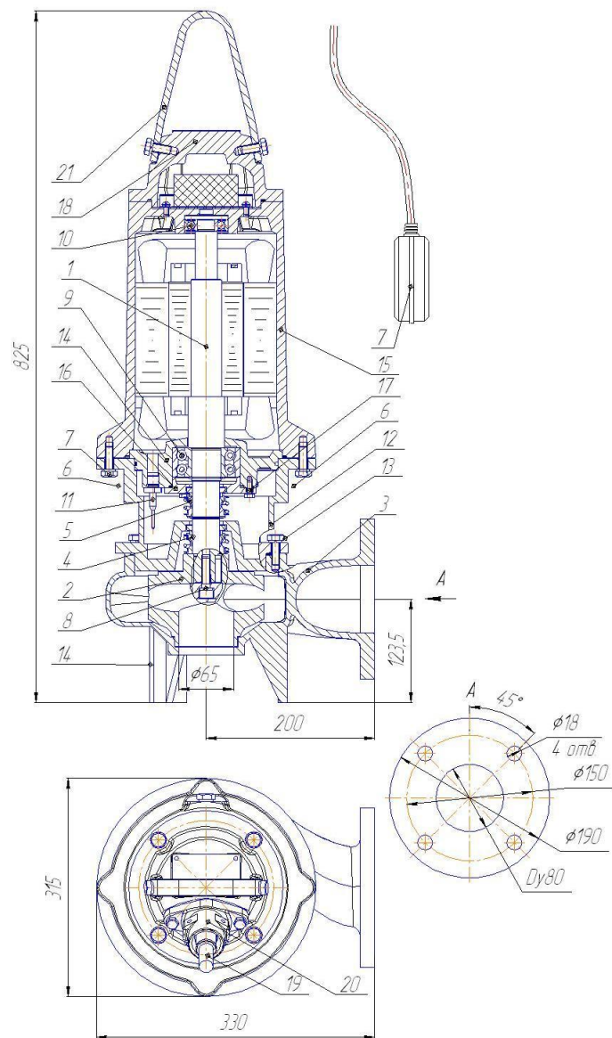
Рис. 37 Общий вид, габаритные и присоединительные размеры электронасоса "Иртыш" ПФ2 80/140 – 5,5/2.
