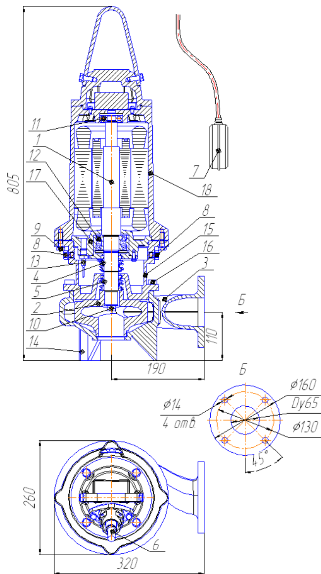
Рис. 25 Общий вид, габаритные и присоединительные размеры электронасоса "Иртыш" ПФ2 65/150 – 5,5/2
