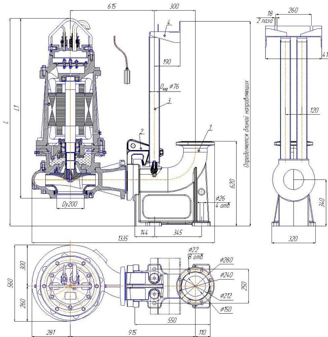
Рис. 104 Общий вид и габаритные размеры электронасоса "Иртыш" ПФ2 150/315 – 22/6– 106; ПФ2 150/315 – 37/4– 106; ПФ2 150/315 – 45/4– 106; ПФ2 150/315 – 55/4– 106 с опускающим устройством.
