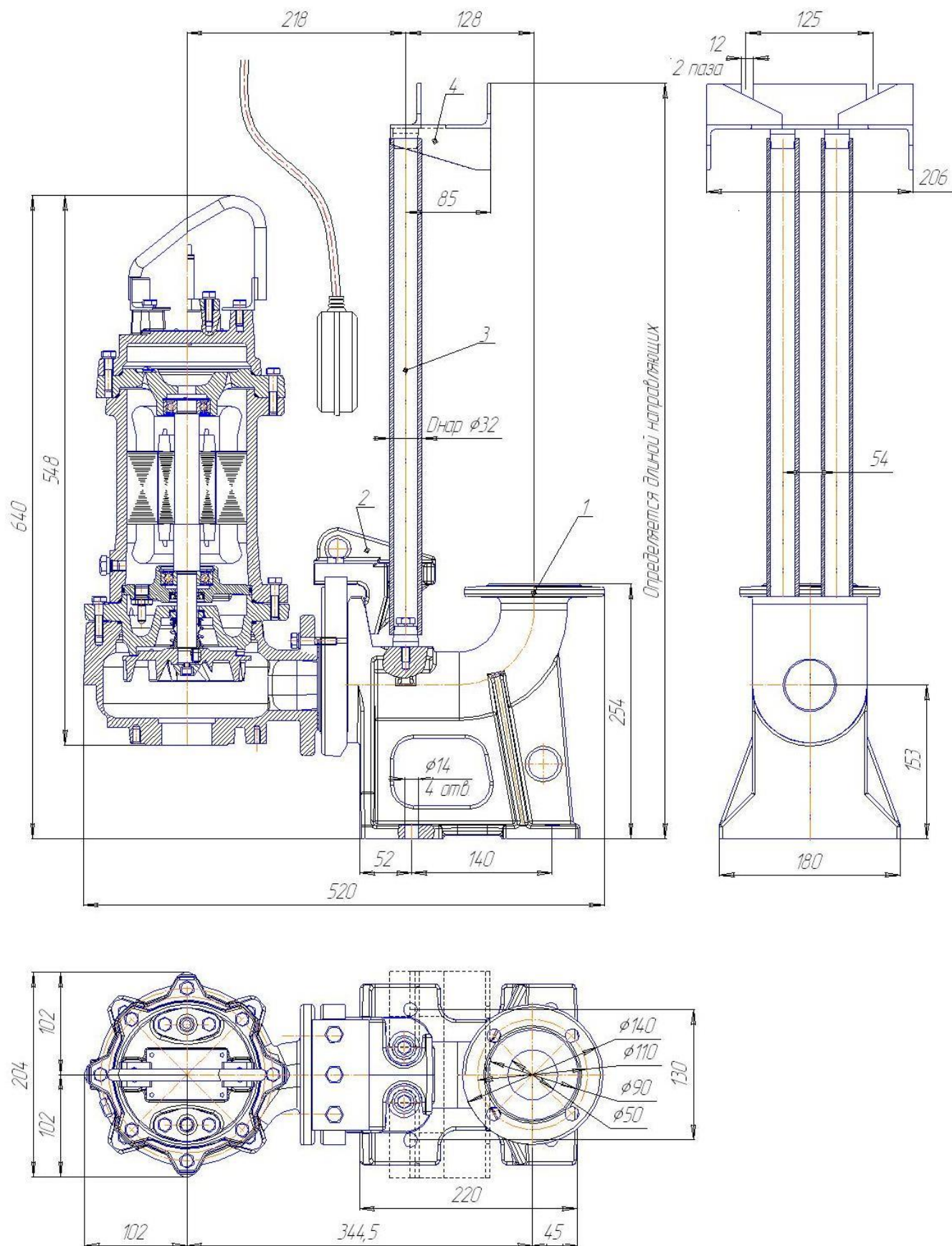
Рис. 65 Общий вид и габаритные размеры электронасоса "Иртыш" ПФс 50/125 – 1,1/2 – 106; ПФс 50/125 – М1,1/2 – 106; ПФ2 50/125 – 1,1/2 – 106; ПФ2 50/125 – М1,1/2 – 106 с опускающим устройством.
