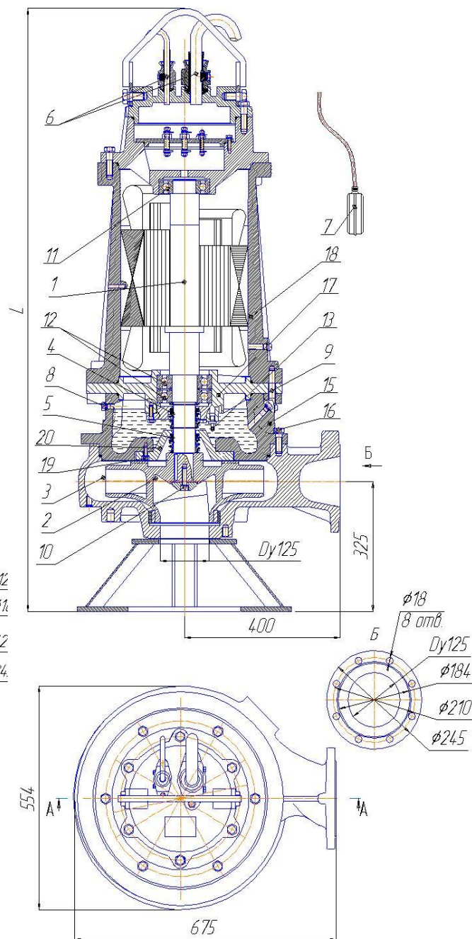
Рис. 50 Общий вид, габаритные и присоединительные размеры электронасоса "Иртыш" ПФ2 125/400 – 22/6; ПФ2 125/400 – 37/4; ПФ2 125/400 – 45/4; ПФ2 125/400 – 55/4.
