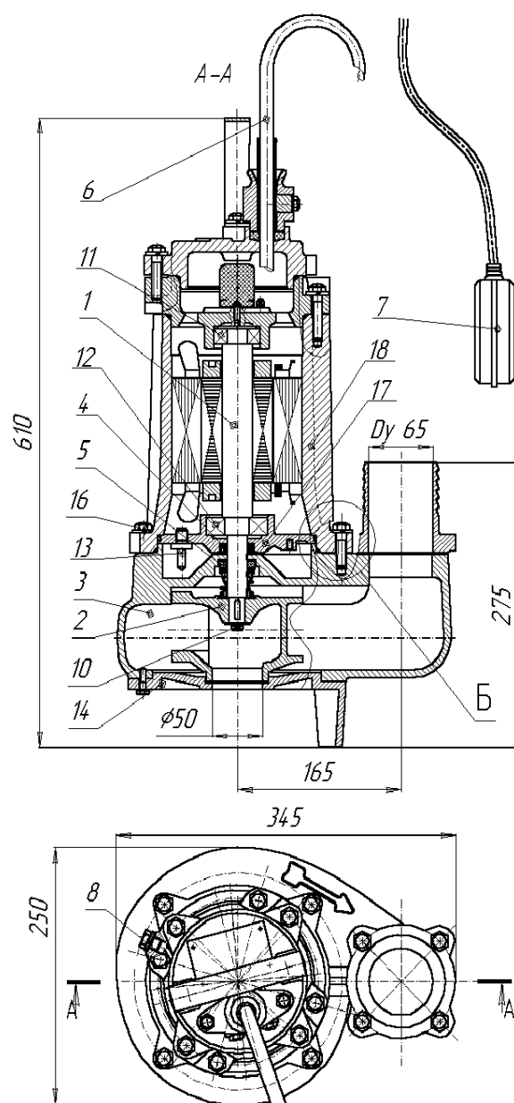
Рис. 27 Общий вид, габаритные и присоединительные размеры электронасоса "Иртыш" ПФ1 65/160 – 3/2; ПФс 65/160 – 3/2;
