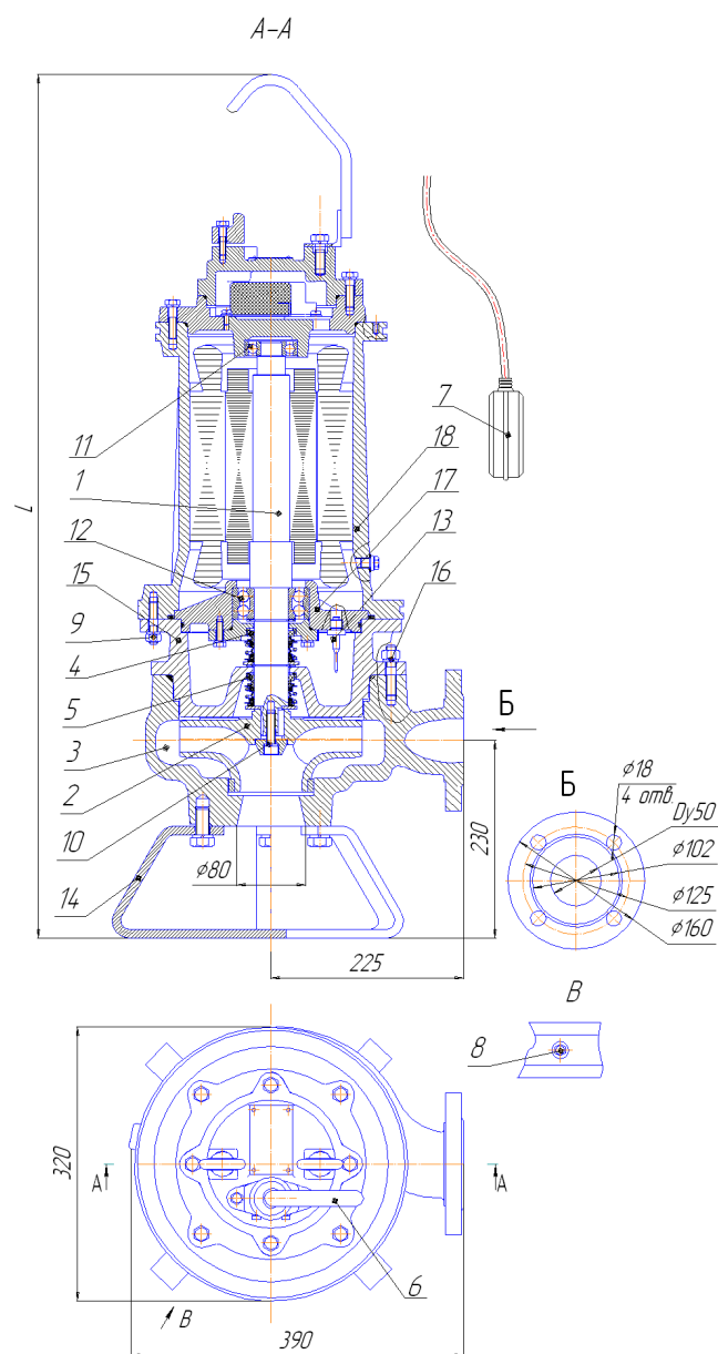
Рис. 21 Общий вид, габаритные и присоединительные размеры электронасоса "Иртыш" ПФ2 50/200 –7,5/2; ПФ2 50/200 –11/2.
