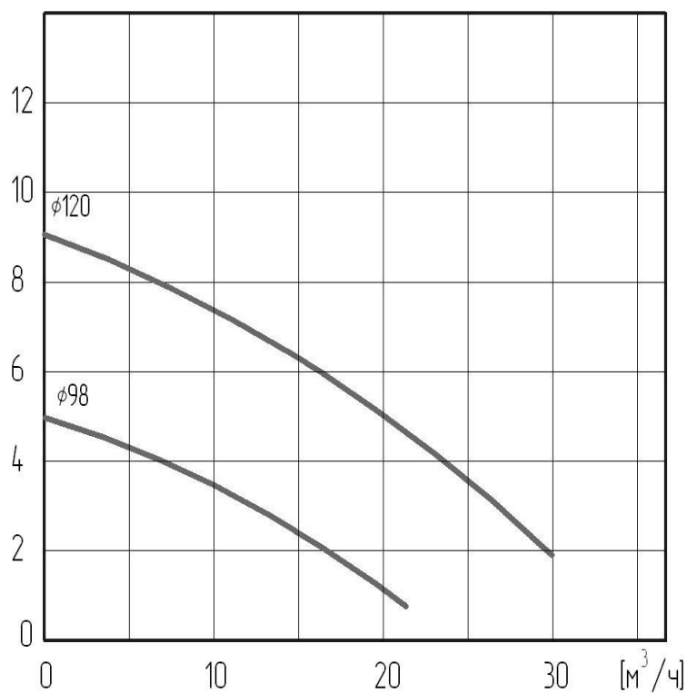
Рис. 1 Рабочие характеристики насоса «Иртыш»: ПФс 50/125.120 – 1,1/2; ПФс 50/125.120 – М1,1/2; ПФс 50/125.98 – 1,1/2; ПФс 50/125.98 – М1,1/2
