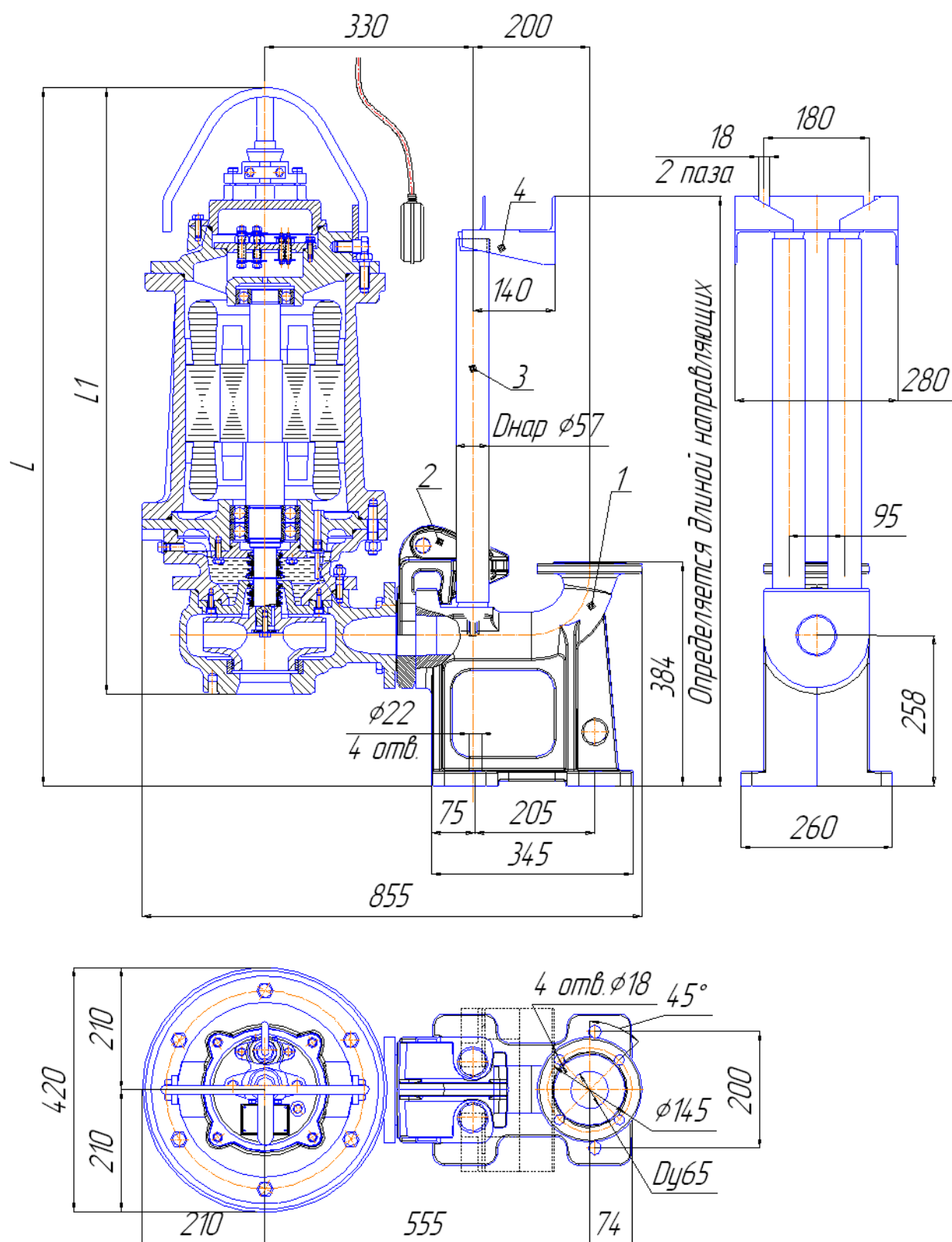
Рис. 84 Общий вид и габаритные размеры электронасоса "Иртыш"
