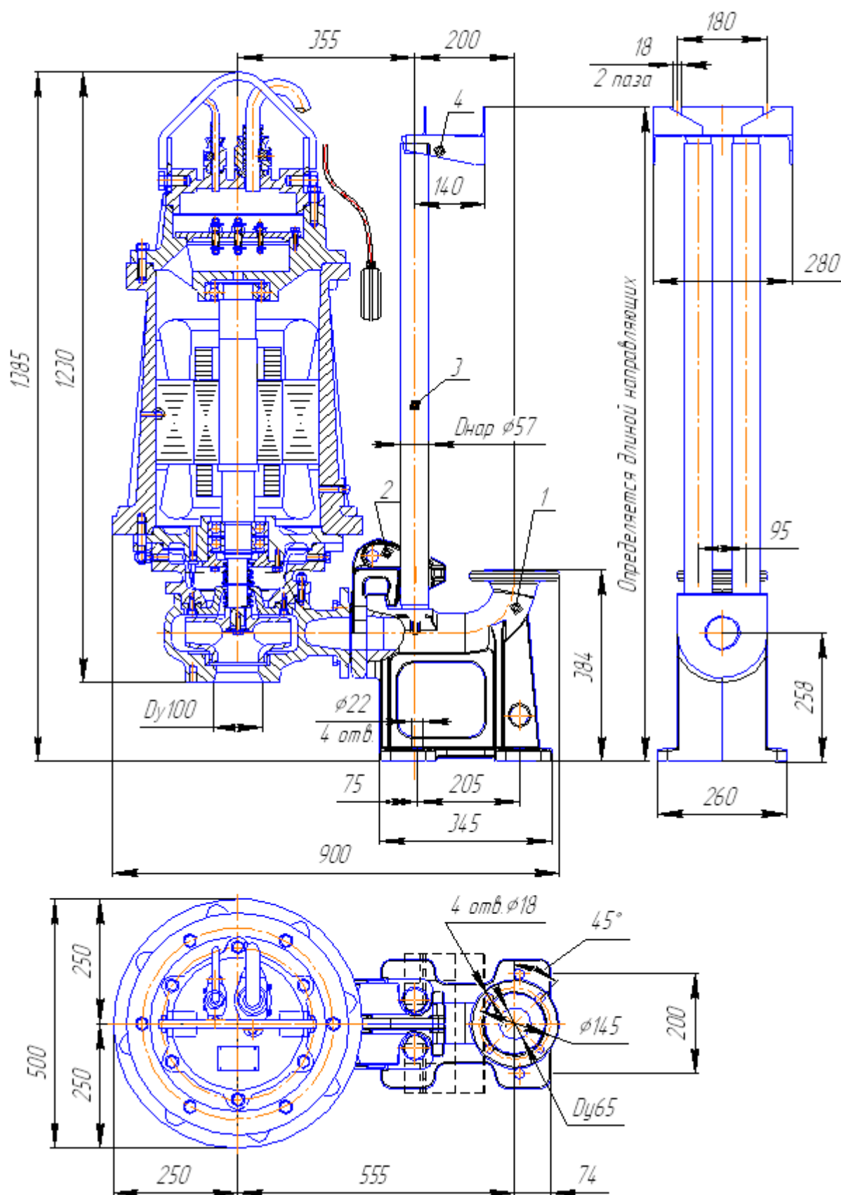
Рис. 85 Общий вид и габаритные размеры электронасоса "Иртыш" ПФ2 65/200 – 37/2 – 106 с опускным устройством.
