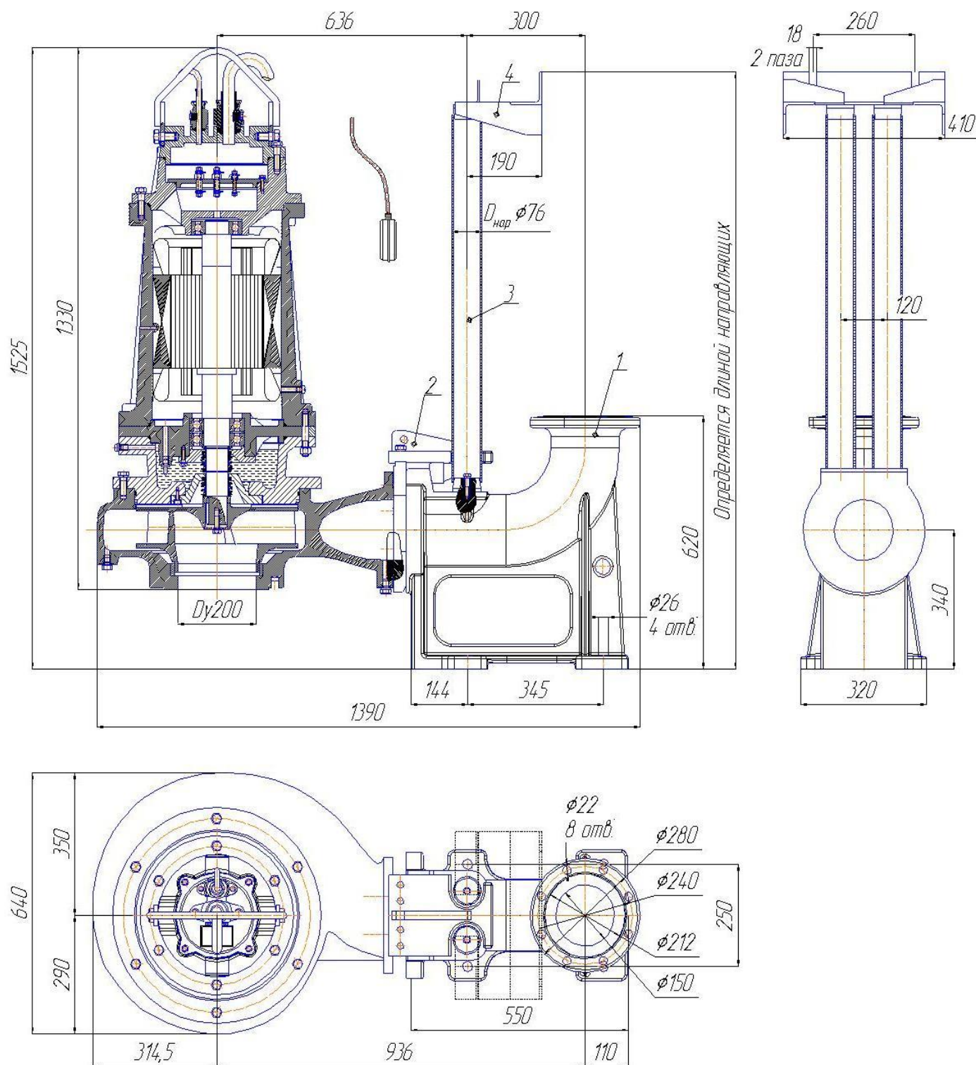
Рис. 106 Общий вид и габаритные размеры электронасоса "Иртыш" ПФ3 150/400 – 22/6– 106; ПФ3 150/400 – 30/6 – 106 с опускающим устройством.
