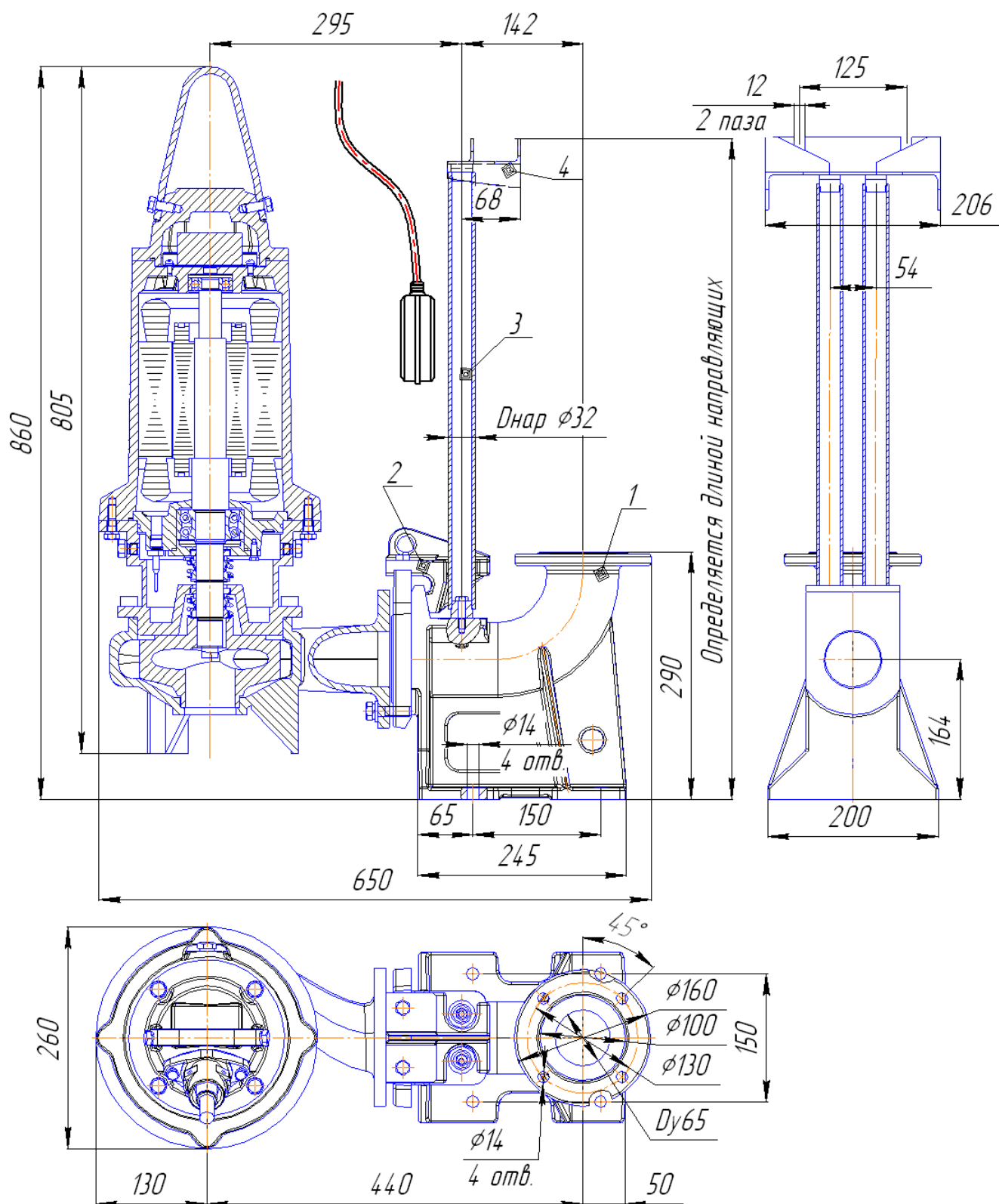
Рис. 73 Общий вид и габаритные размеры электронасоса "Иртыш" ПФ2 65/150 – 5,5/2 – 106 с опускающим устройством.
