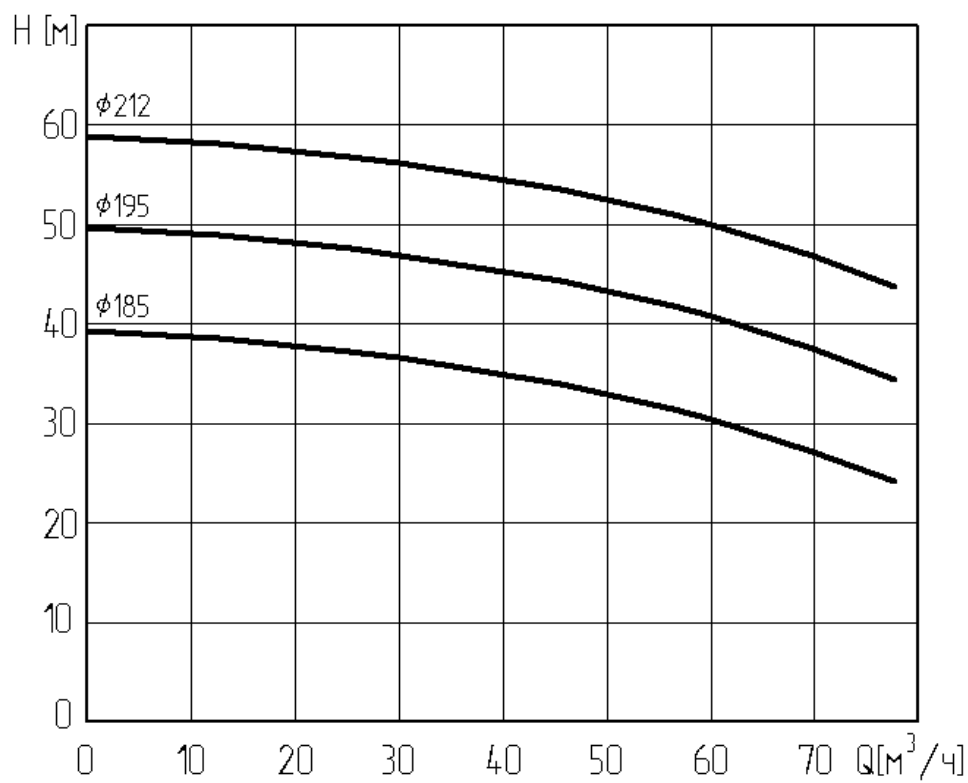
Рис. 2 Рабочие характеристики насоса «Иртыш»: ПФ2 50/200.185 – 11/2 ПФ2 50/200.195 – 15/2 ПФ2 50/200.212 – 18,5/2
