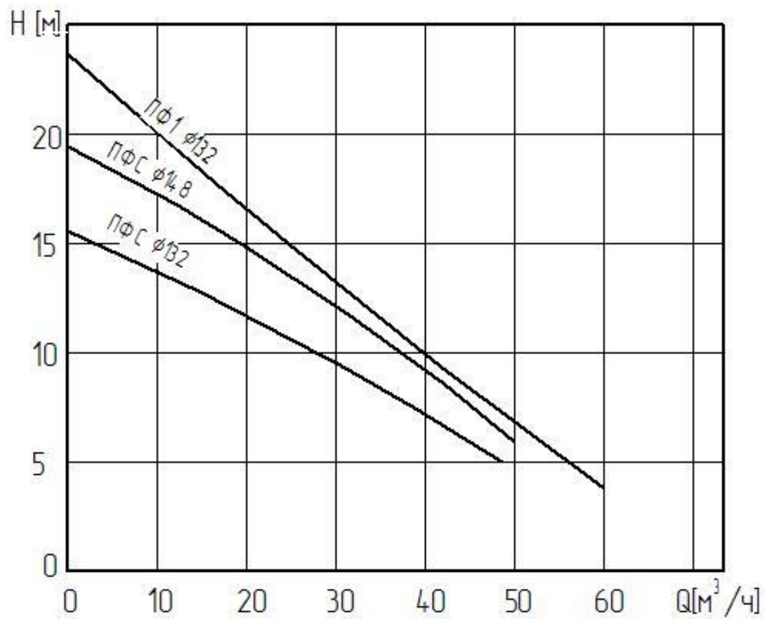
Рис. 3 Рабочие характеристики насоса «Иртыш»: ПФС 65/160.132 – 3/2, ПФС 65/160.148 – 3/2, ПФ1 65/160.132 – 3/2
