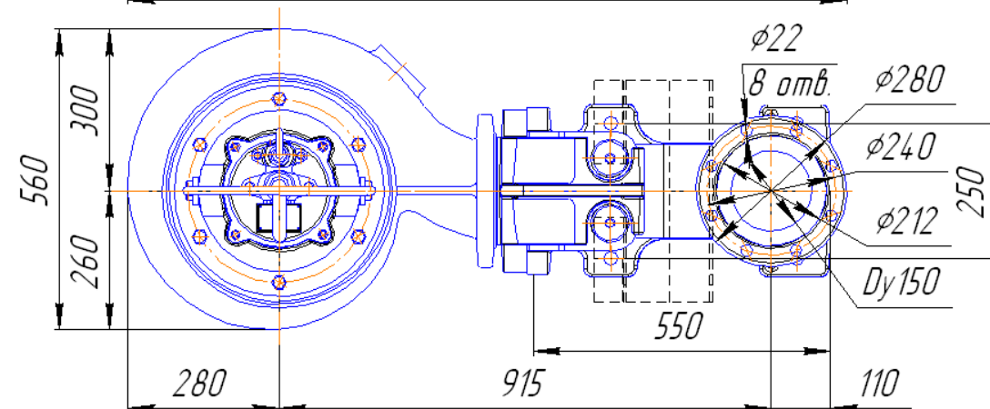
Рис. 103 Общий вид и габаритные размеры электронасоса "Иртыш" ПФ2 150/315 – 11/6– 106; ПФ2 150/315 – 15/6– 106; ПФ2 150/315 – 18,5/6– 106 с опускающим устройством.
