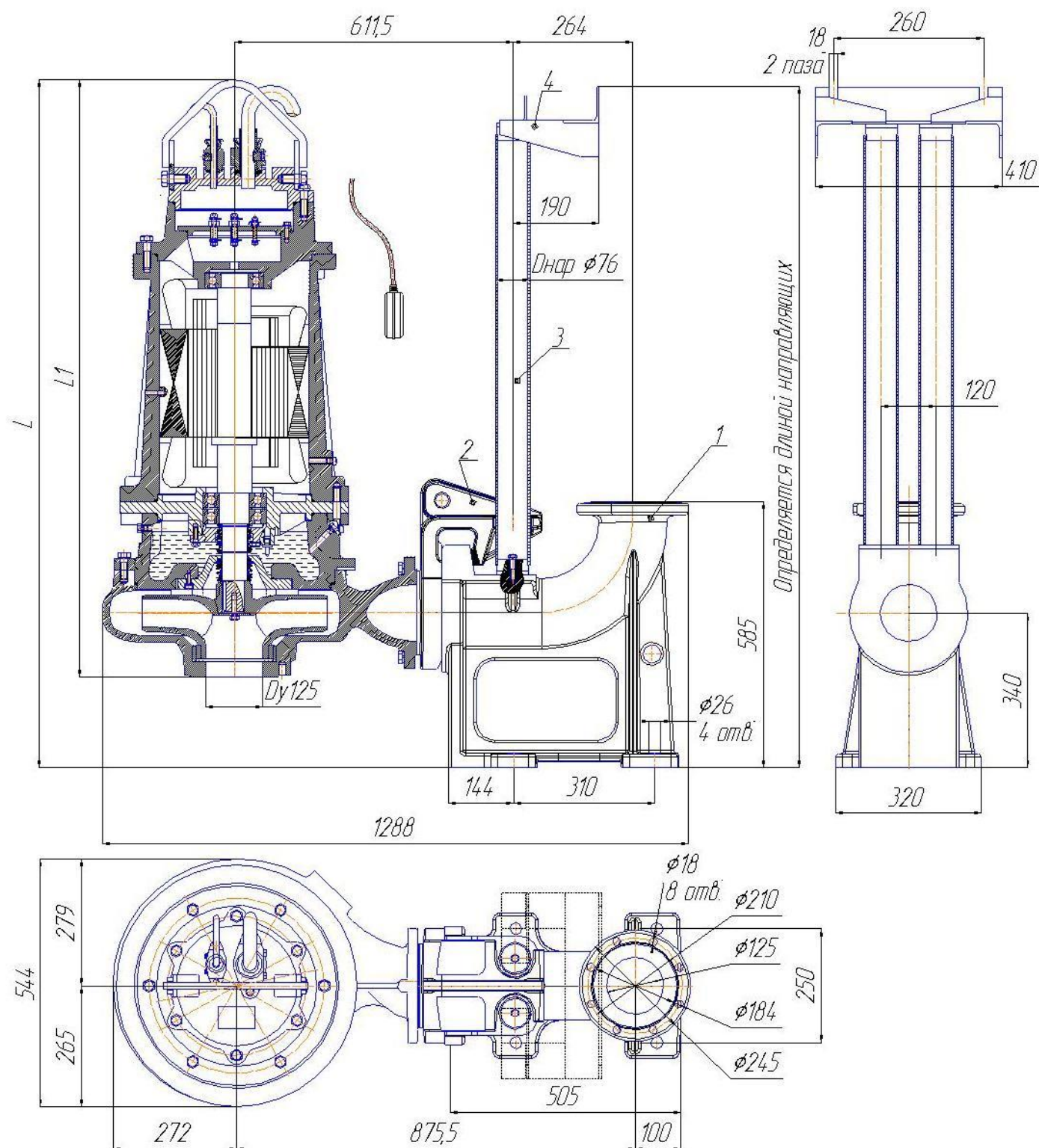
Рис. 99 Общий вид и габаритные размеры электронасоса "Иртыш"
