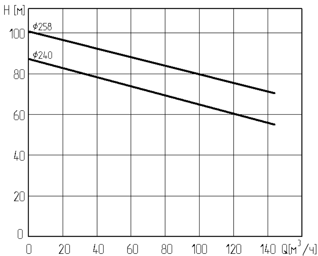
Рис. 5 Рабочие характеристики насоса «Иртыш»:
