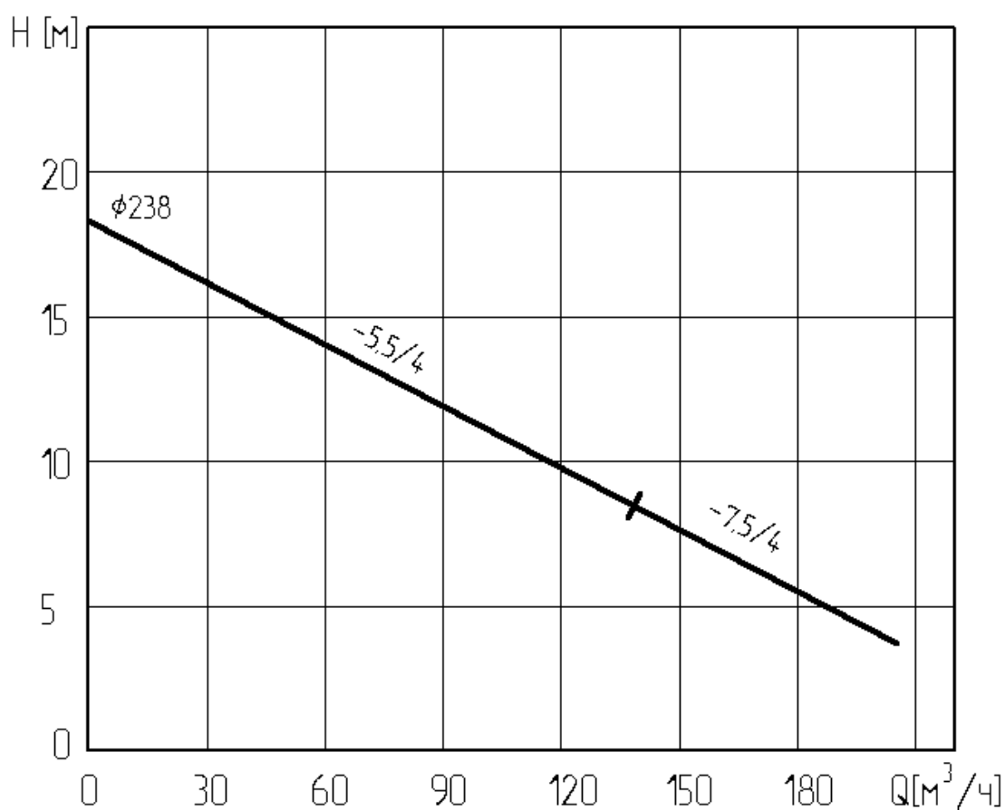
Рис. 8 Рабочие характеристики насоса «Иртыш»: ПФ1 100/240.238 – 5,5/4 ПФ1 100/240.238 – 7,5/4
