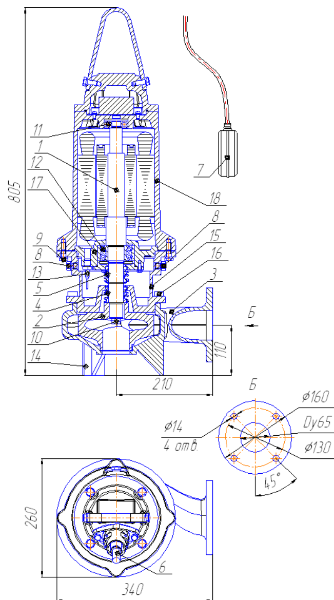
Рис. 29 Общий вид, габаритные и присоединительные размеры электронасоса "Иртыш" ПФ2 65/165 – 4/2; ПФ2 65/165 – 5,5/2;
