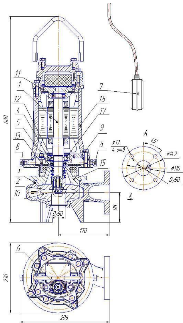
Рис.18 Общий вид, габаритные и присоединительные размеры электронасоса "Иртыш" ПФ2 50/140. – 3/2
