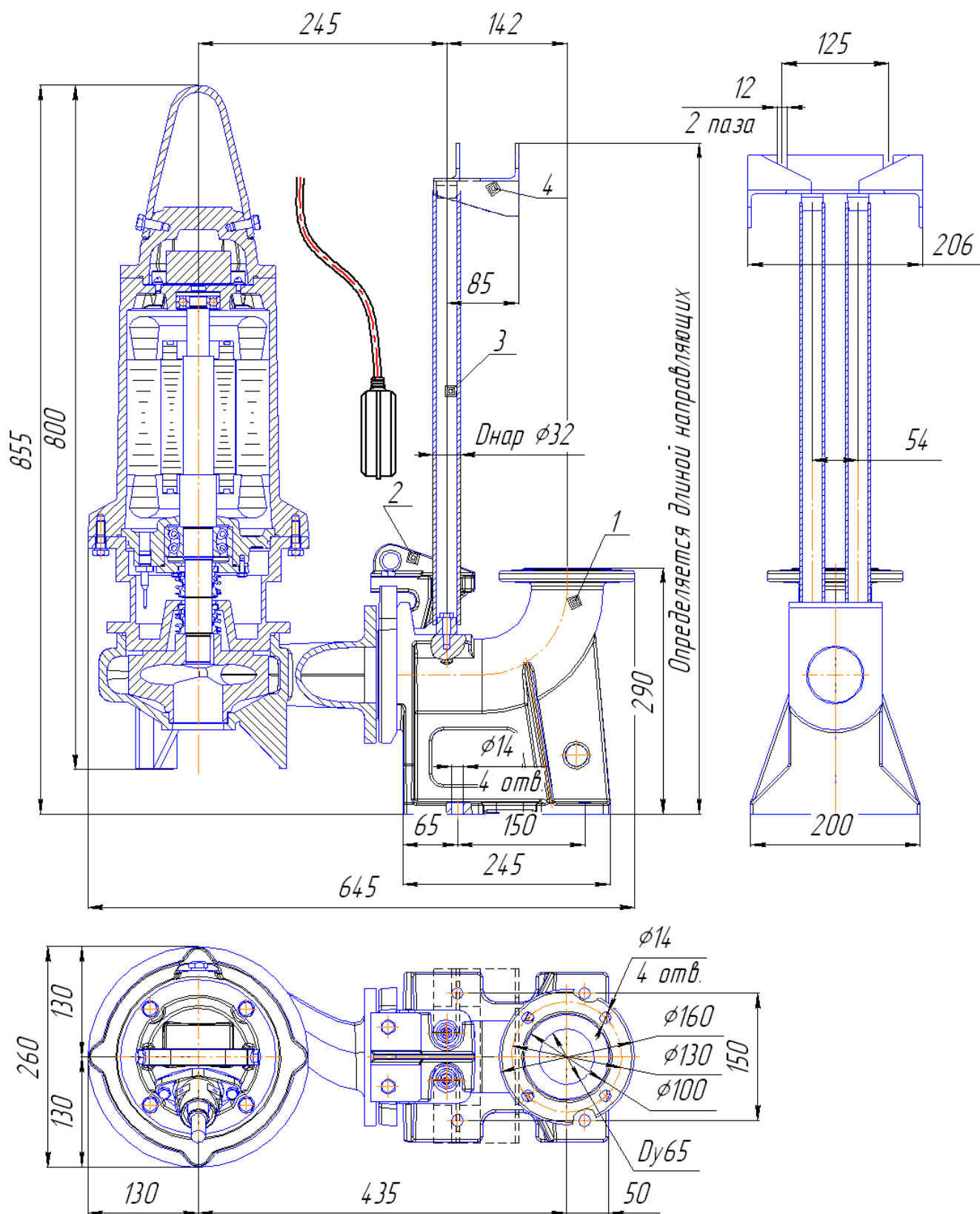
Рис. 75 Общий вид и габаритные размеры электронасоса "Иртыш" ПФ2 65/155 – 4/2 – 106; ПФ2 65/155 – 5,5/2 – 106 с опускающим устройством
