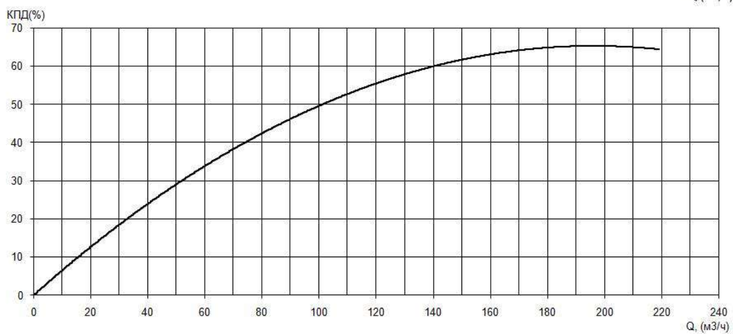
Приложение 1 Рис. 1. Рабочие характеристики электронасоса серии «Иртыш» ЦМЛ 150/225-45/2.
