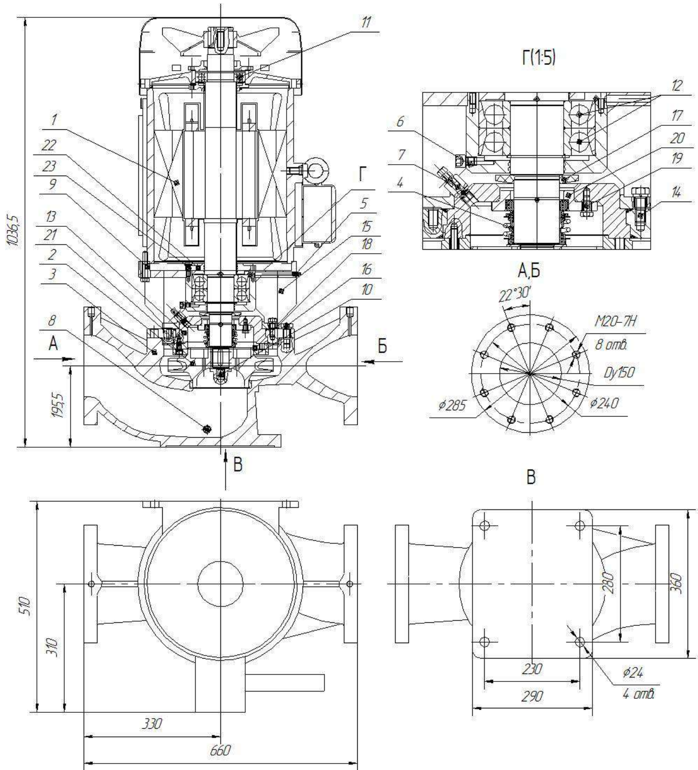
Приложение 1 Рис. 2. Общий вид, габаритные и присоединительные размеры электронасоса серии «Иртыш» ЦМЛ 150/225-45/2.
