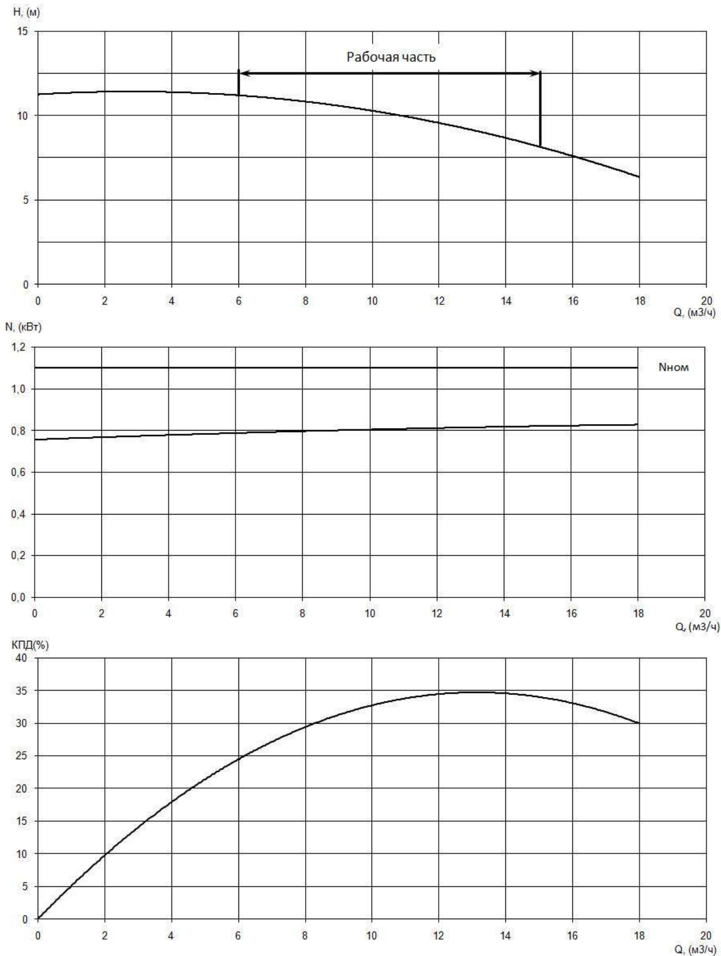
Приложение 1 Рис. 1. Рабочие характеристики электронасоса «Иртыш» ЦМЛ 50/95-1,1/2.
