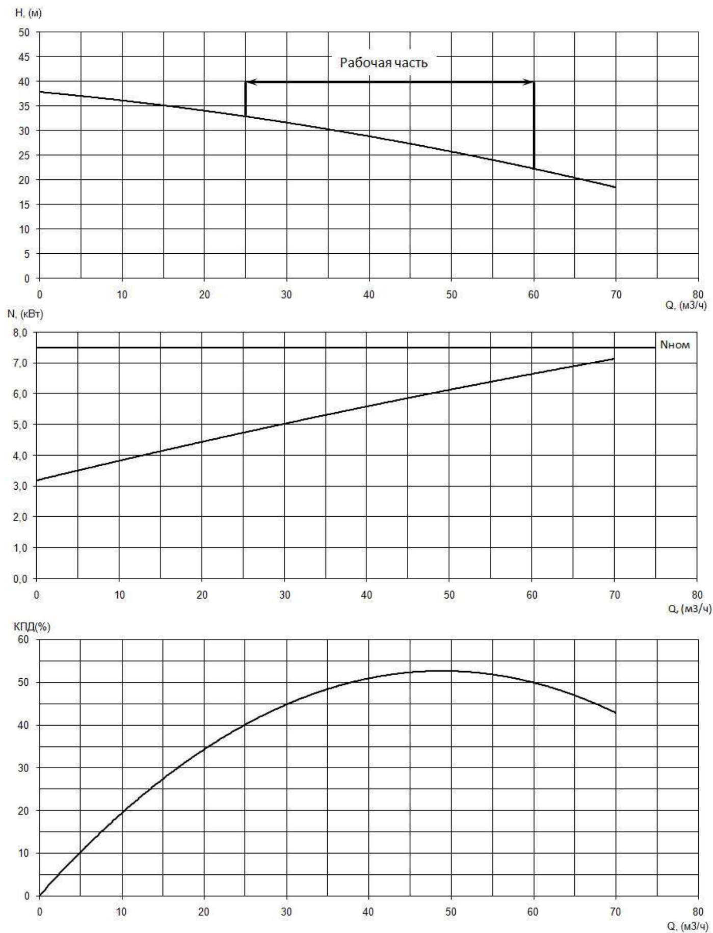
Приложение 1 Рис. 1. Рабочие характеристики электронасоса серии «Иртыш» ПФ2 65/165.157-7,5/2.
