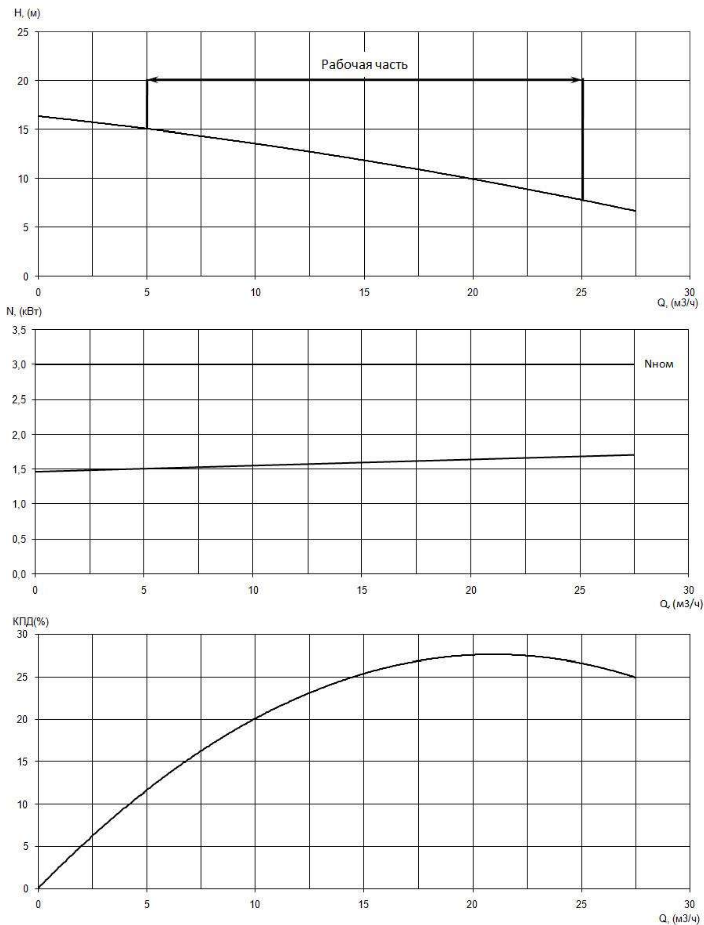
Приложение 1. Рис. 1. Рабочие характеристики электронасоса серии «Иртыш» ПФс 50/140.130-3/2.
