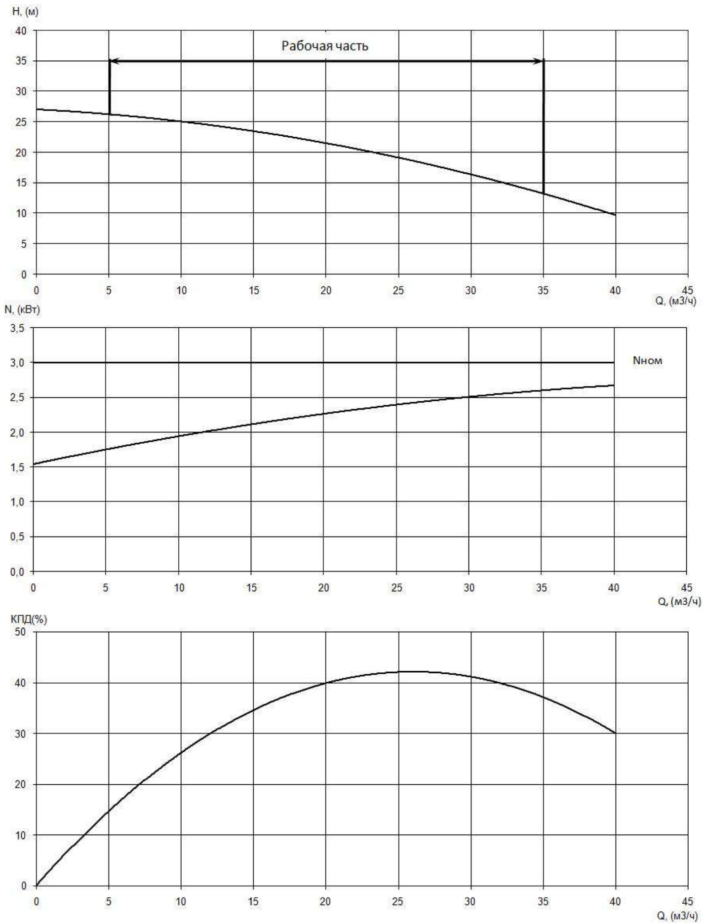
Приложение 1 Рис.1. Рабочие характеристики электронасоса серии «Иртыш» ПФс 50/150.154-3/2.
