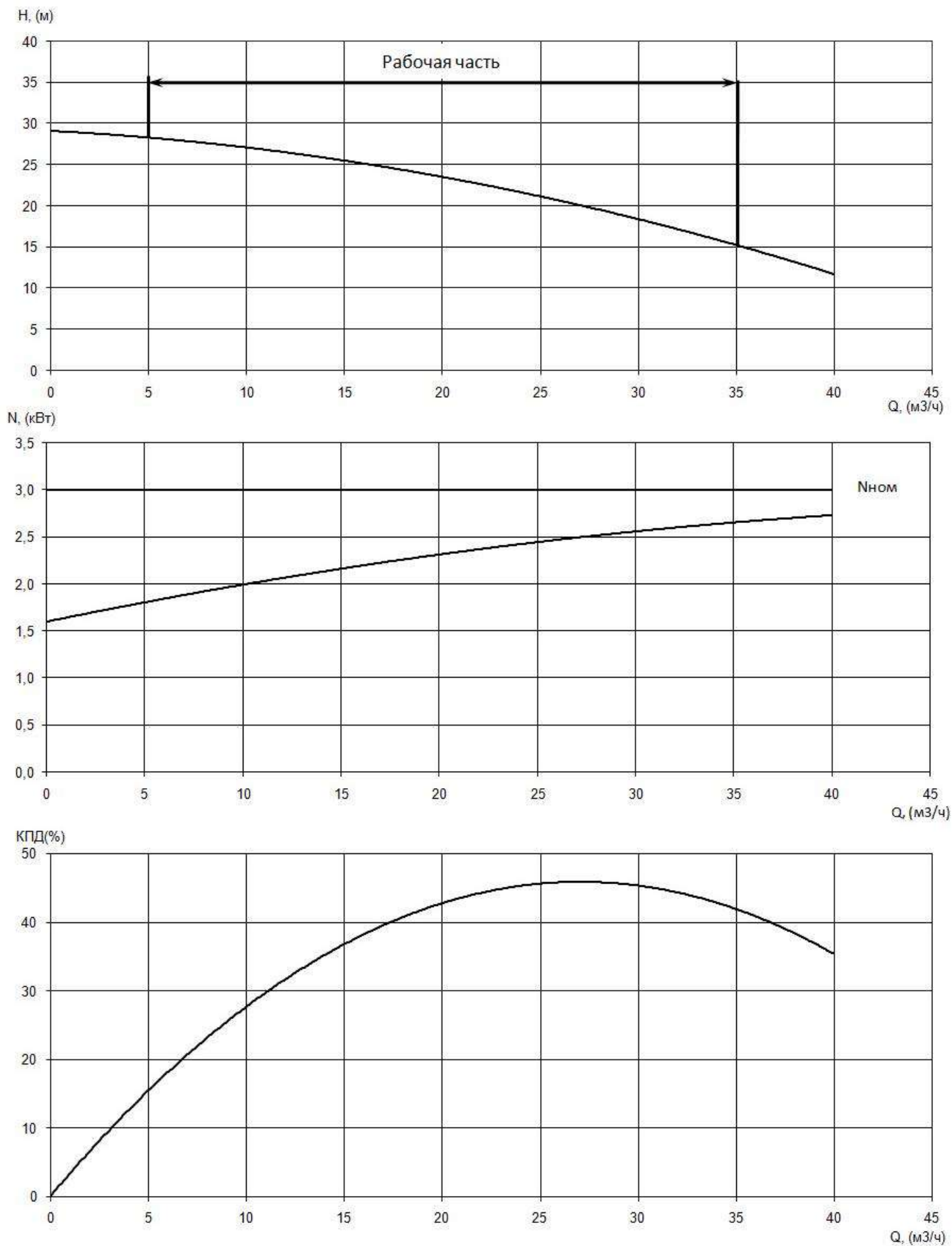
Приложение 1 Рис.1. Рабочие характеристики электронасоса серии «Иртыш» ПФс 50/150.156-3/2.
