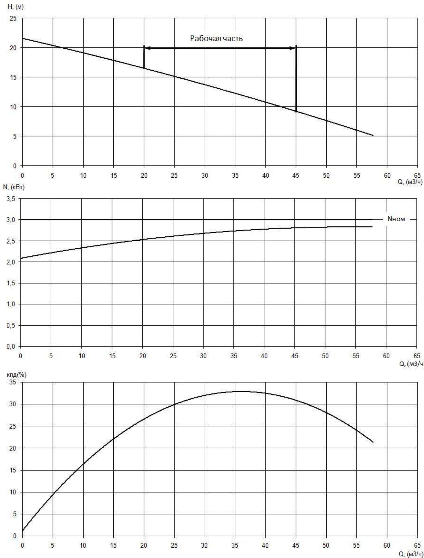
Приложение 1. Рис. 1 Рабочие характеристики электронасоса серии «Иртыш» ПФс 65/160.150-3/2.
