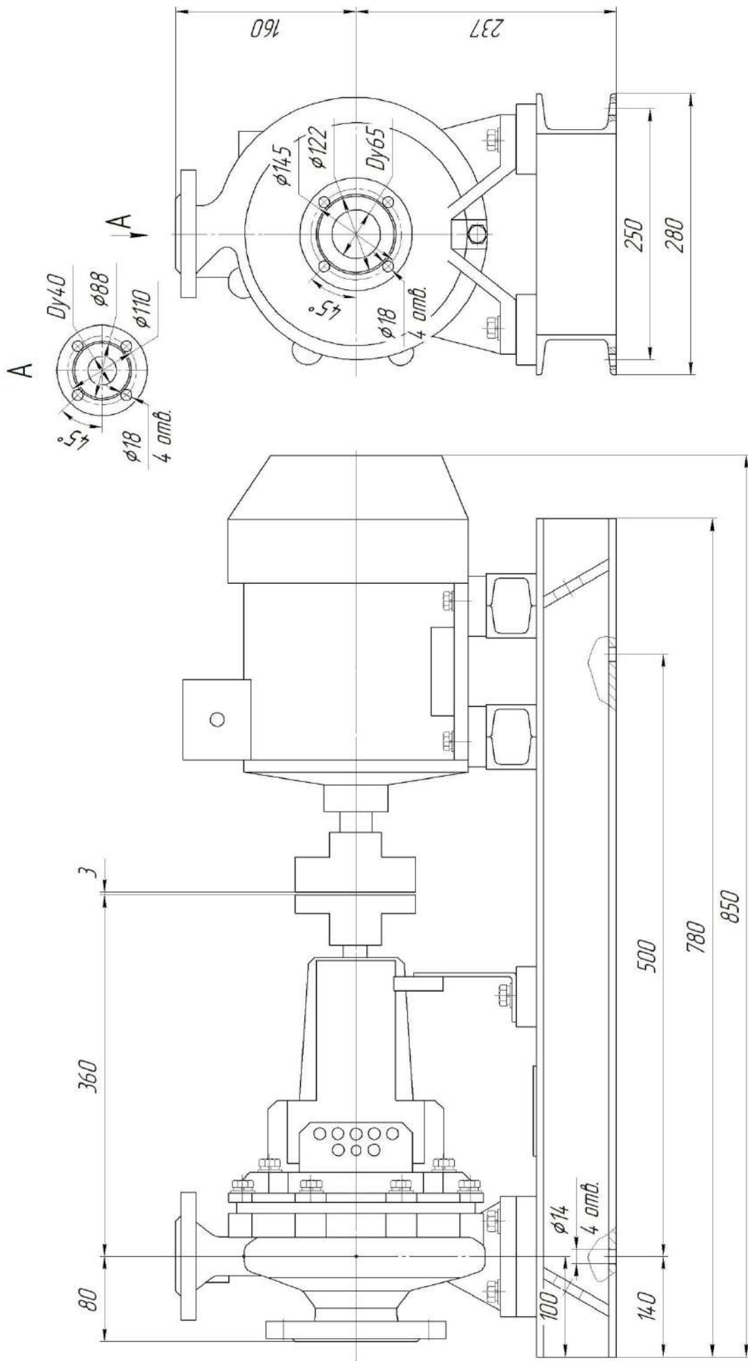
Приложение 1 Рис. 2. Общий вид, габаритные присоединительные размеры электронасоса серии «Иртыш» ЦНК 40/160.155.08-5,5/2-400.
