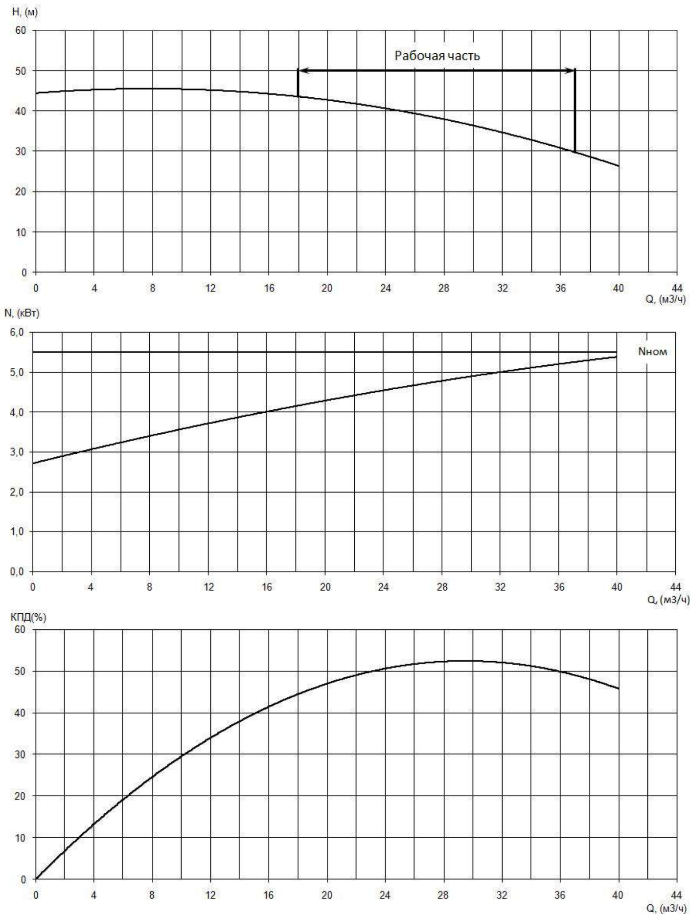
Приложение 1 Рис. 1. Рабочие характеристики электронасоса серии «Иртыш» ЦНК 40/160.155.08-5,5/2.
