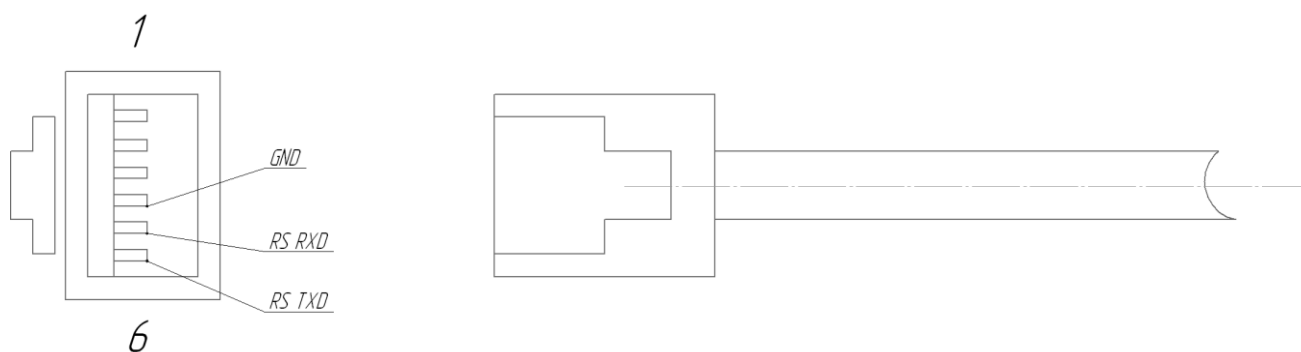
Рисунок 2. Разъем RJ12
