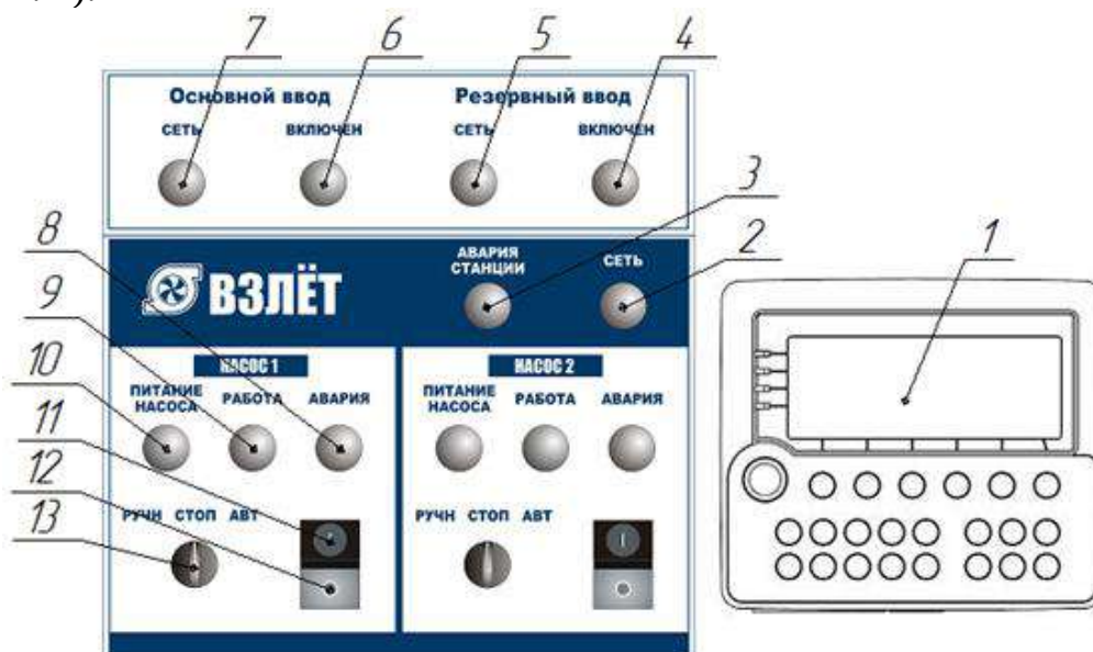
Рисунок 1 – Органы управления и индикации шкафа управления
