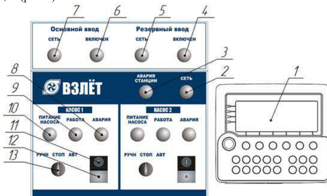
Рисунок 1 – Органы управления и индикации шкафа управления
