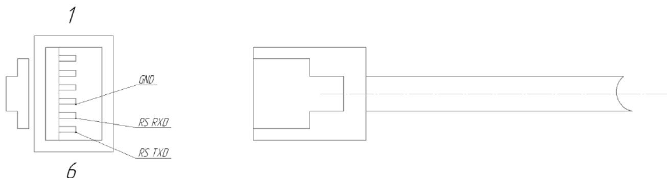
Рисунок 2. Разъем RJ12
