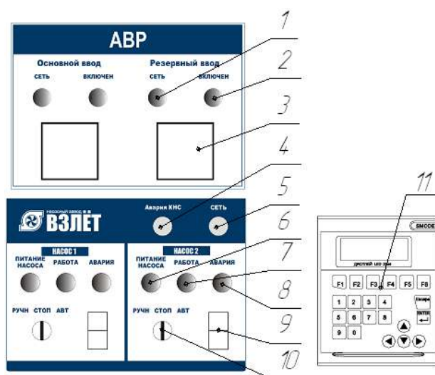
Рисунок 1 – Органы управления и индикации шкафа управления
