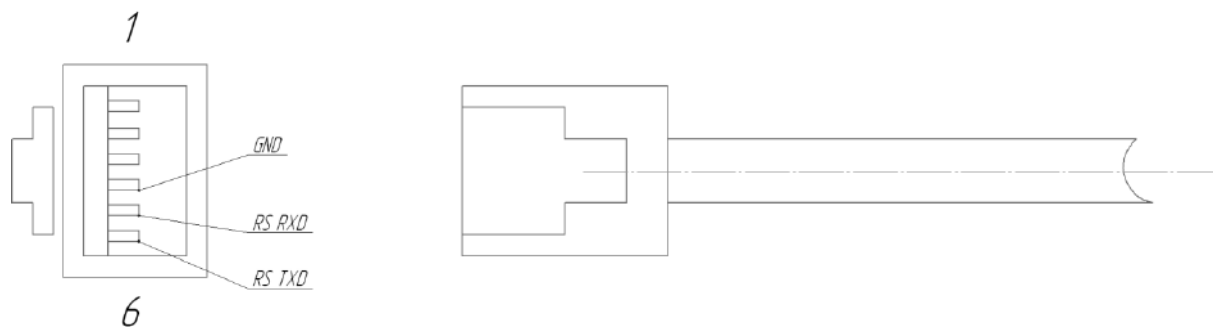
Рисунок 2. Разъем RJ12
