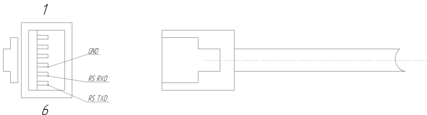
Рисунок 2. Разъем RJ12
