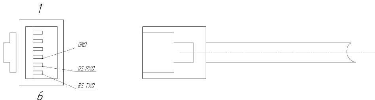
Рисунок 2. Разъем RJ12
