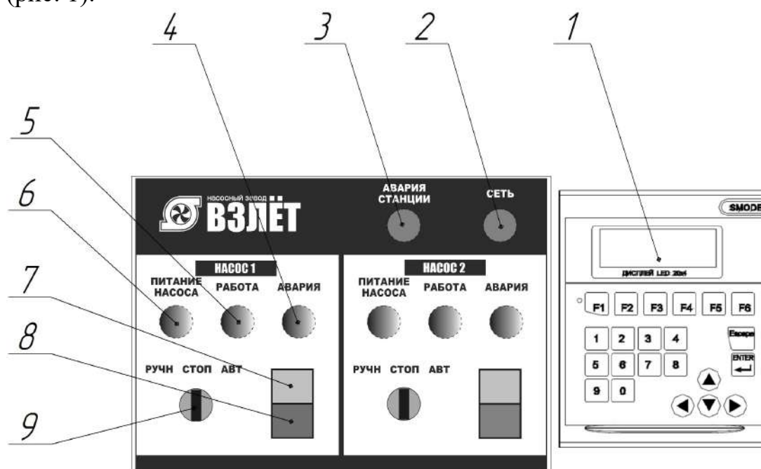
Рисунок 1 – Органы управления и индикации шкафа управления
