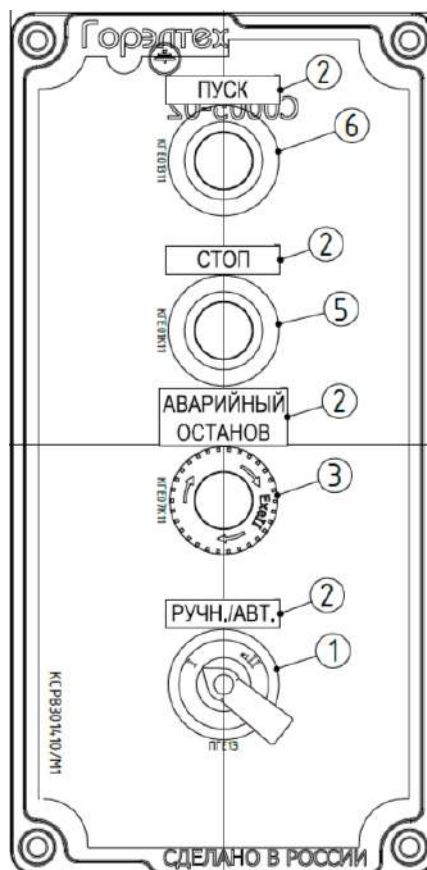
Рисунок 2 - Общий вид кнопочного поста
