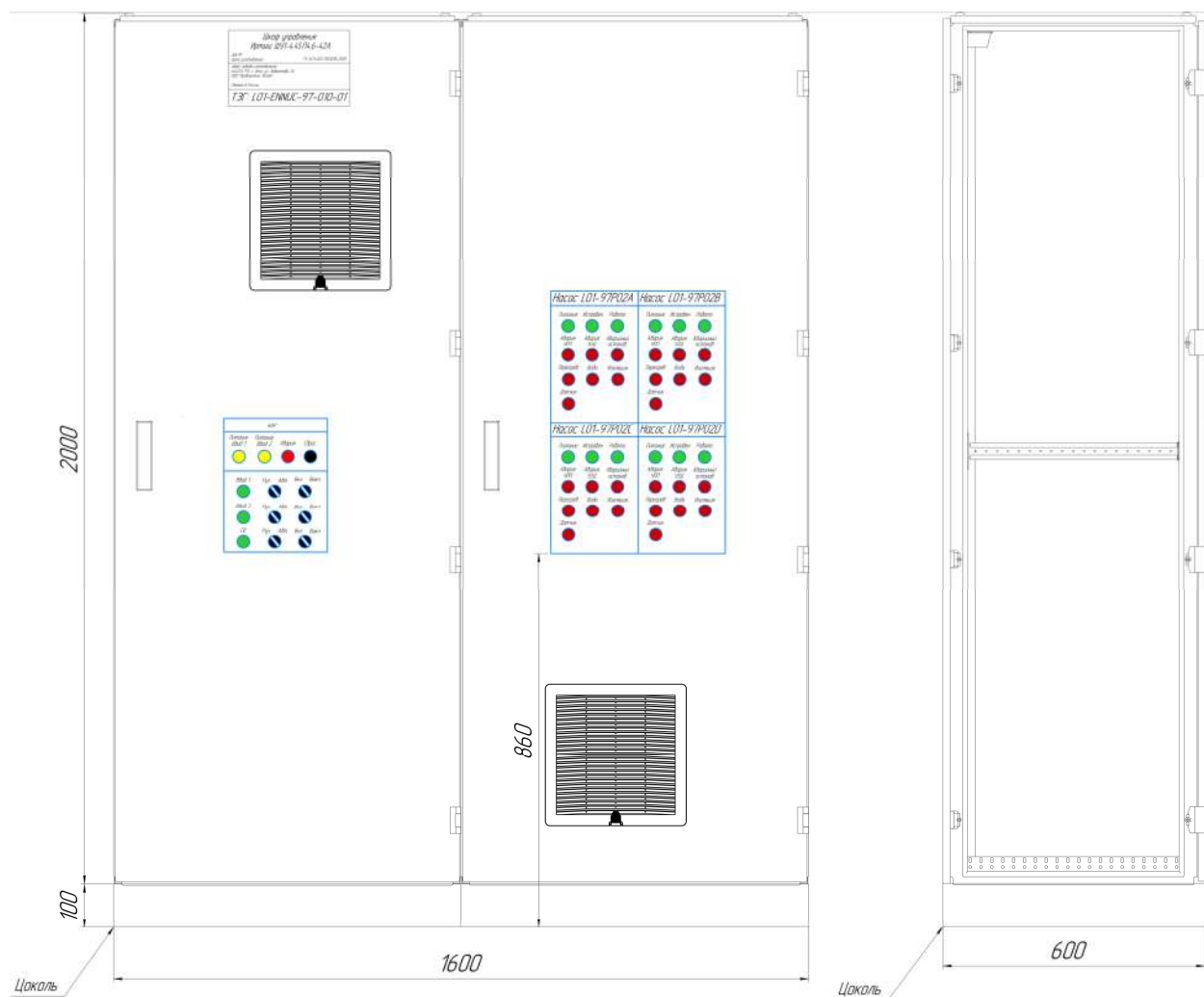
Рисунок 3 - Габариты шкафа
