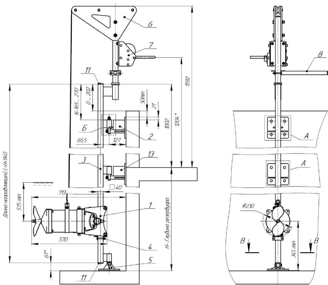
Рис. 1 Общий вид и габариты мешалки "Иртыш" Иртыш ПМ2 230-1,1/8-116
