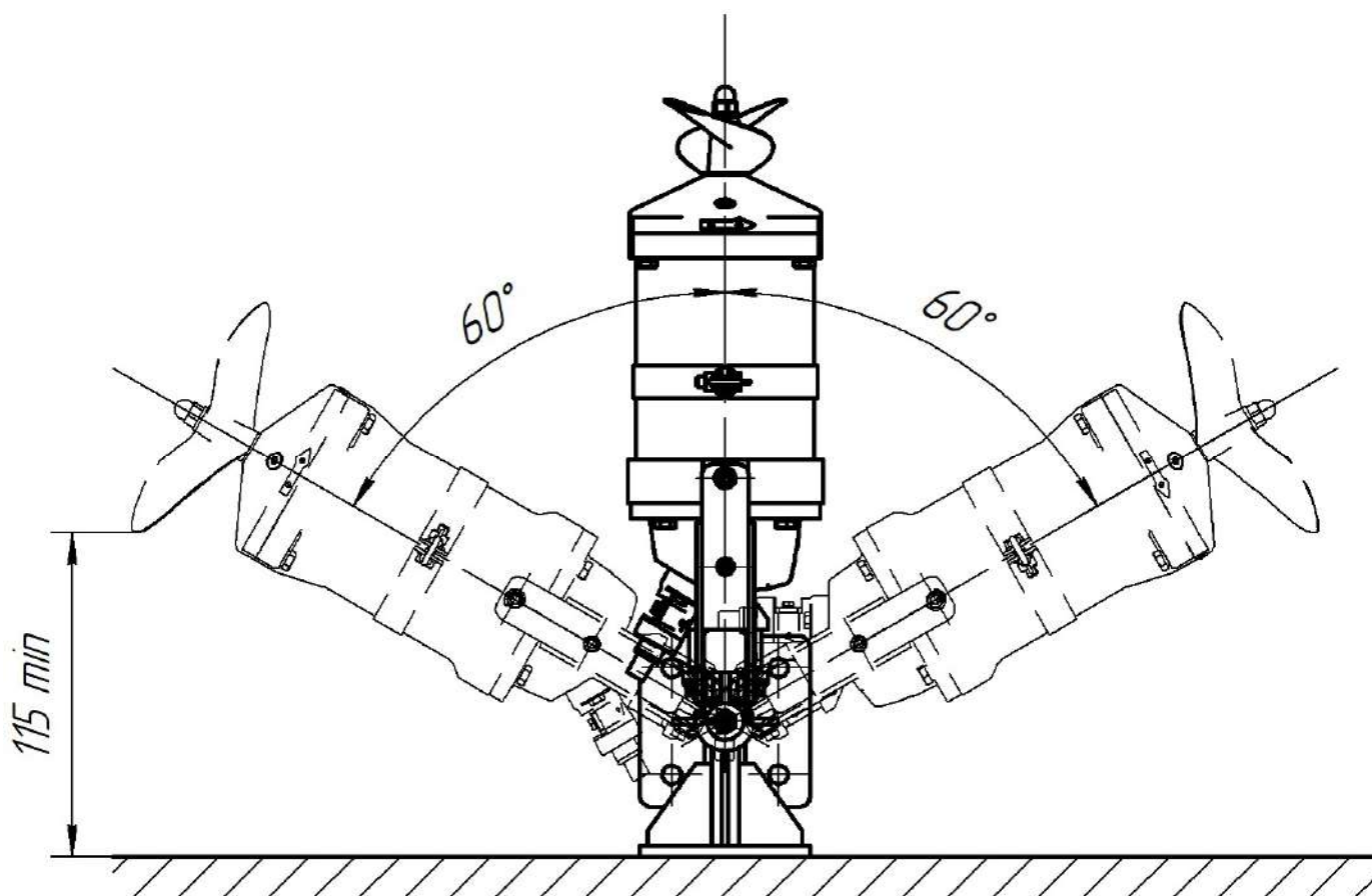
Рис. 2 Углы установки мешалки "Иртыш" ПМ2 230-1,1/8-116 в горизонтальной плоскости.
