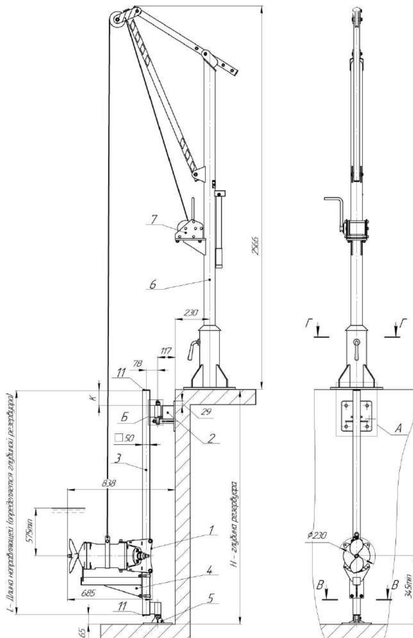
Рис. 1 Общий вид и габариты мешалки "Иртыш" Иртыш ПМ2 230-3/4-116
