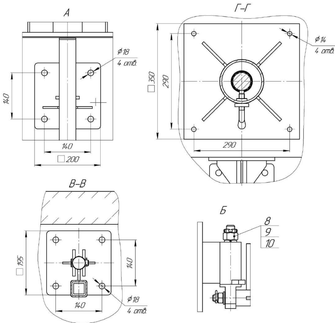
Рис. 1. Общий вид и габариты мешалки "Иртыш" Иртыш ПМ2 230-3/4-116 с опускным устройством и грузоподъемным механизмом.
