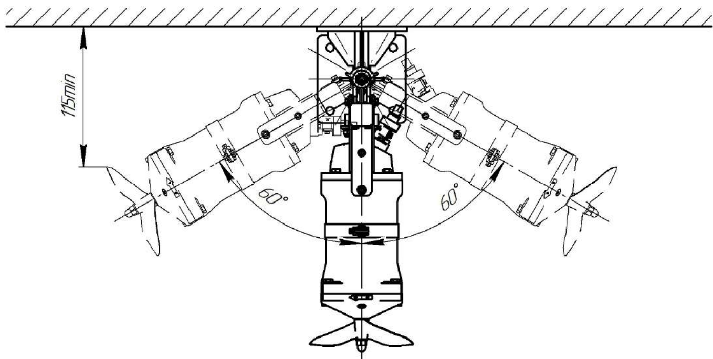
Рис. 2 Углы установки мешалки "Иртыш" ПМ2 230-3/4-116 в горизонтальной плоскости.
