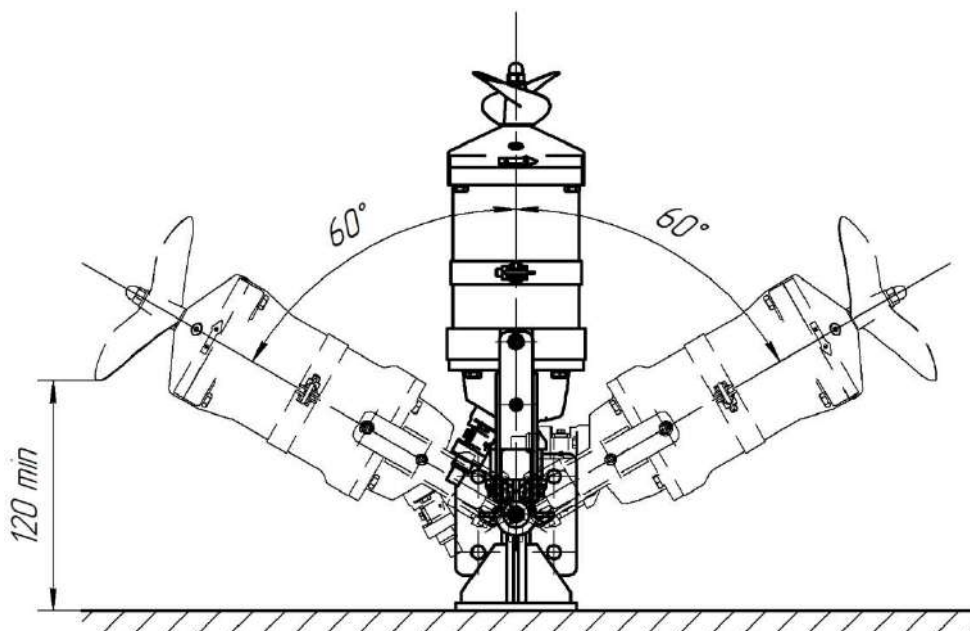
Рис. 2 Углы установки электромешалки "Иртыш" ПМ2 240-1,5/6-116 в горизонтальной плоскости.
