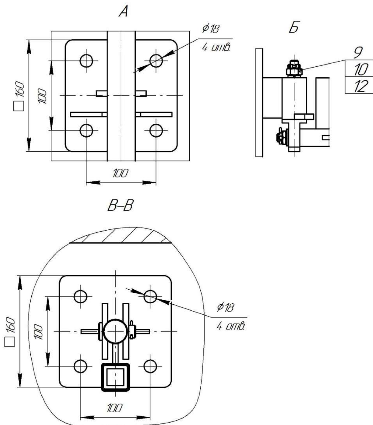
Рис. 1. Общий вид и габариты электромешалки "Иртыш" ПМ2 240-1,5/6-116 с опускным устройством и грузоподъёмным механизмом.
