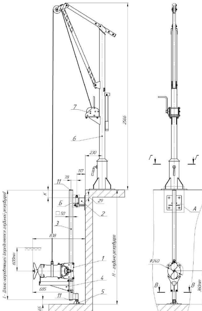
Рис. 1 Общий вид и габариты мешалки "Иртыш" Иртыш ПМ2 240-4/4-116
