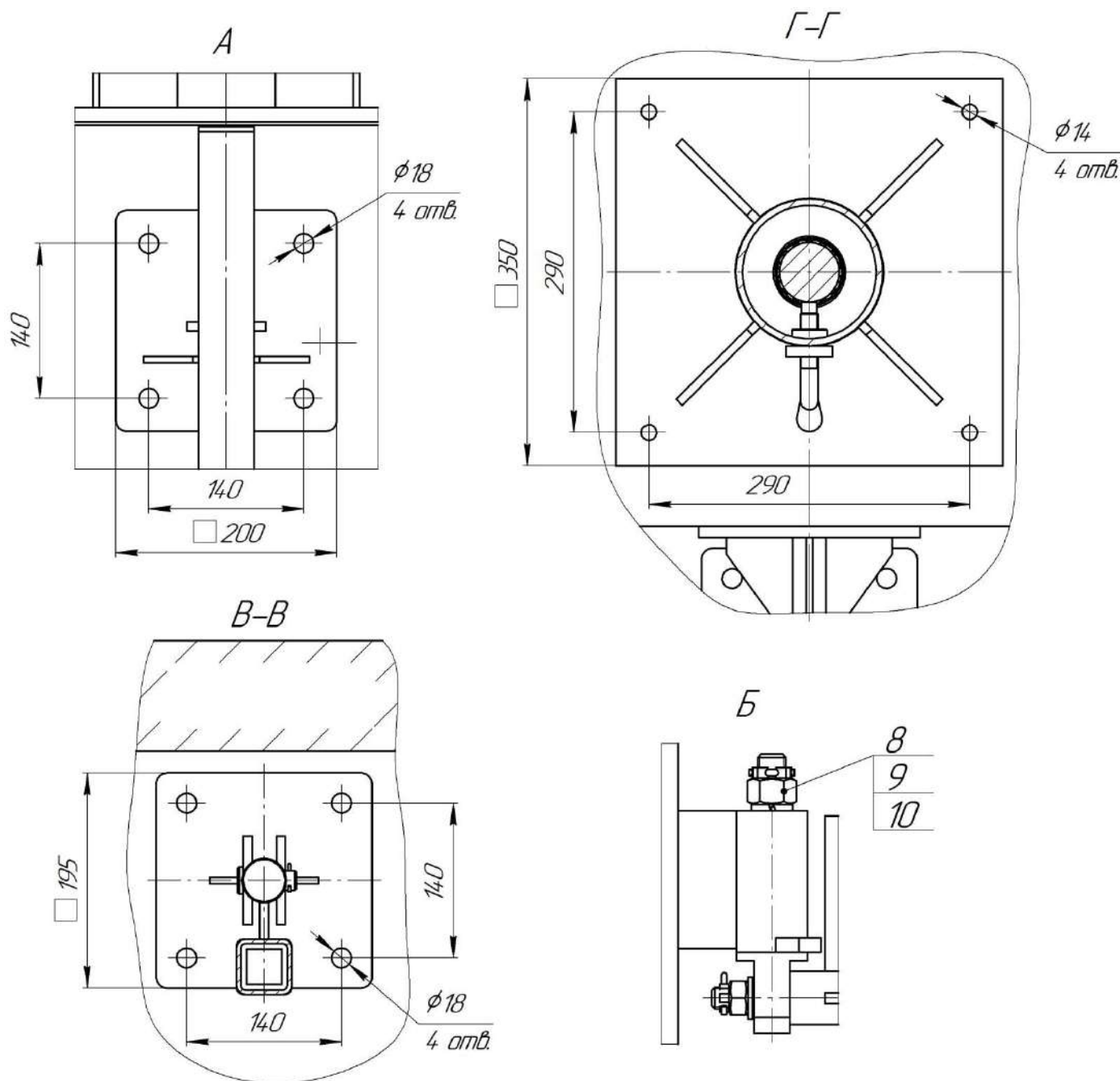
Рис. 1. Общий вид и габариты мешалки "Иртыш" Иртыш ПМ2 240-4/4-116 с опускным устройством и грузоподъемным механизмом.
