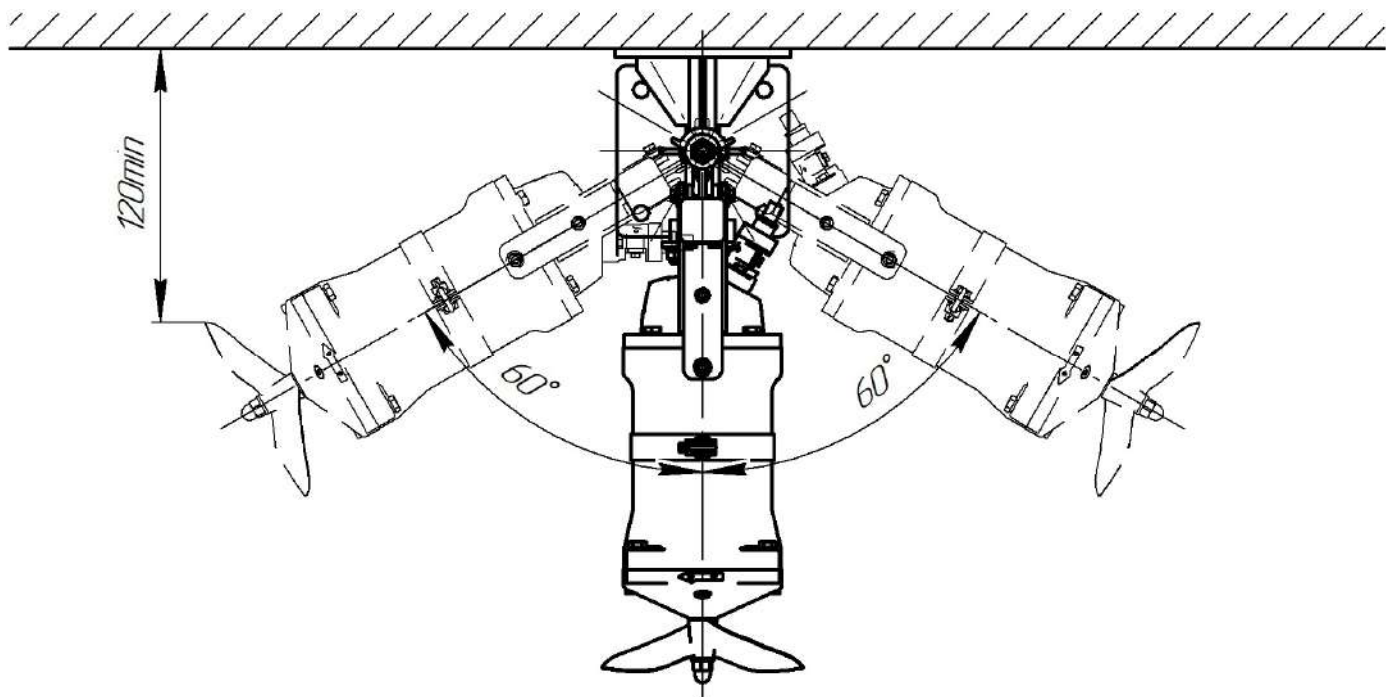
Рис. 2 Углы установки мешалки "Иртыш" ПМ2 240-4/4-116 в горизонтальной плоскости.
