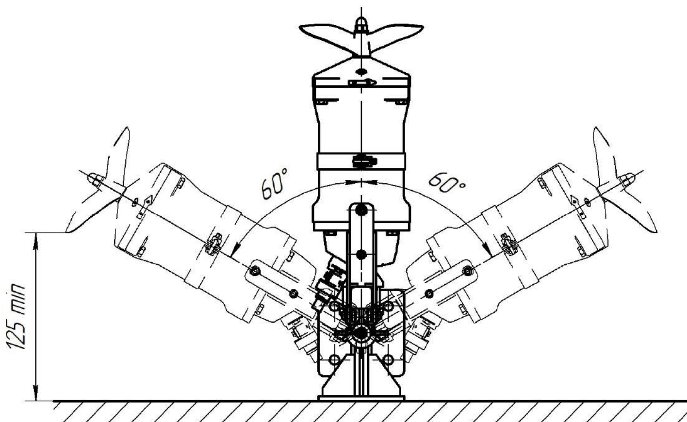
Рис. 2 Углы установки мешалки "Иртыш" ПМ2 250-1,1/6-116 в горизонтальной плоскости.
