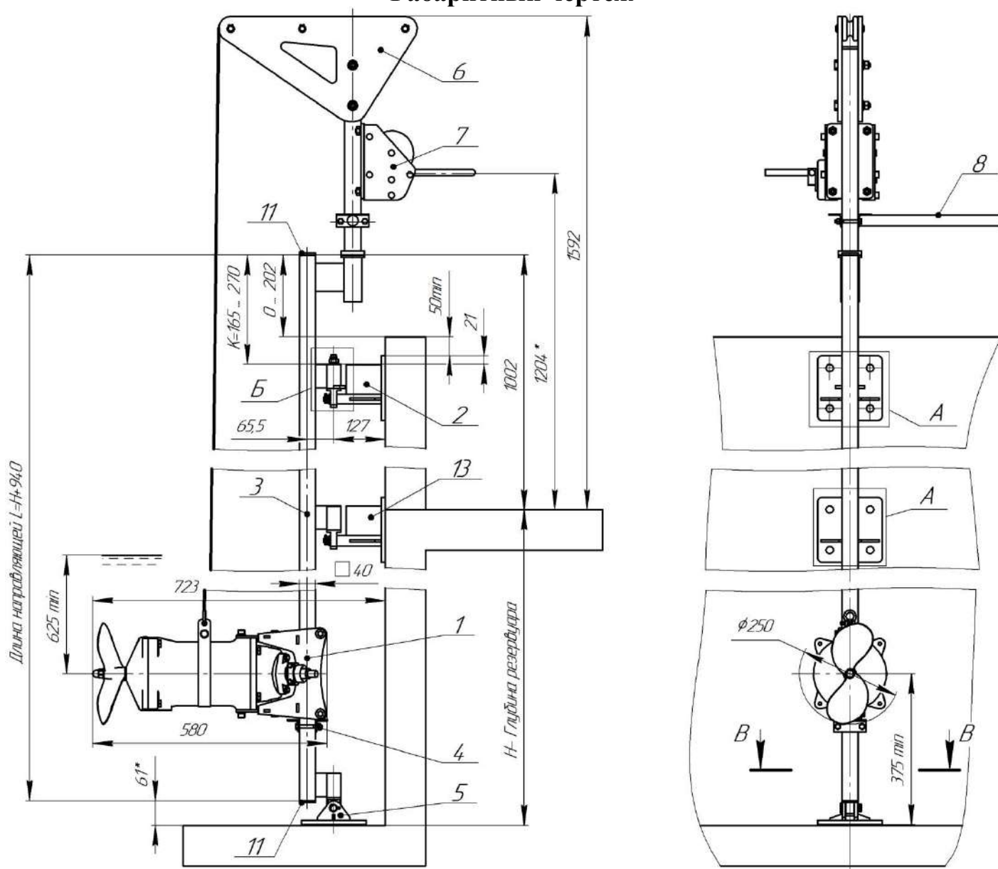
Рис. 1 Общий вид и габариты мешалки "Иртыш" Иртыш ПМ2 250-1,1/6-116
