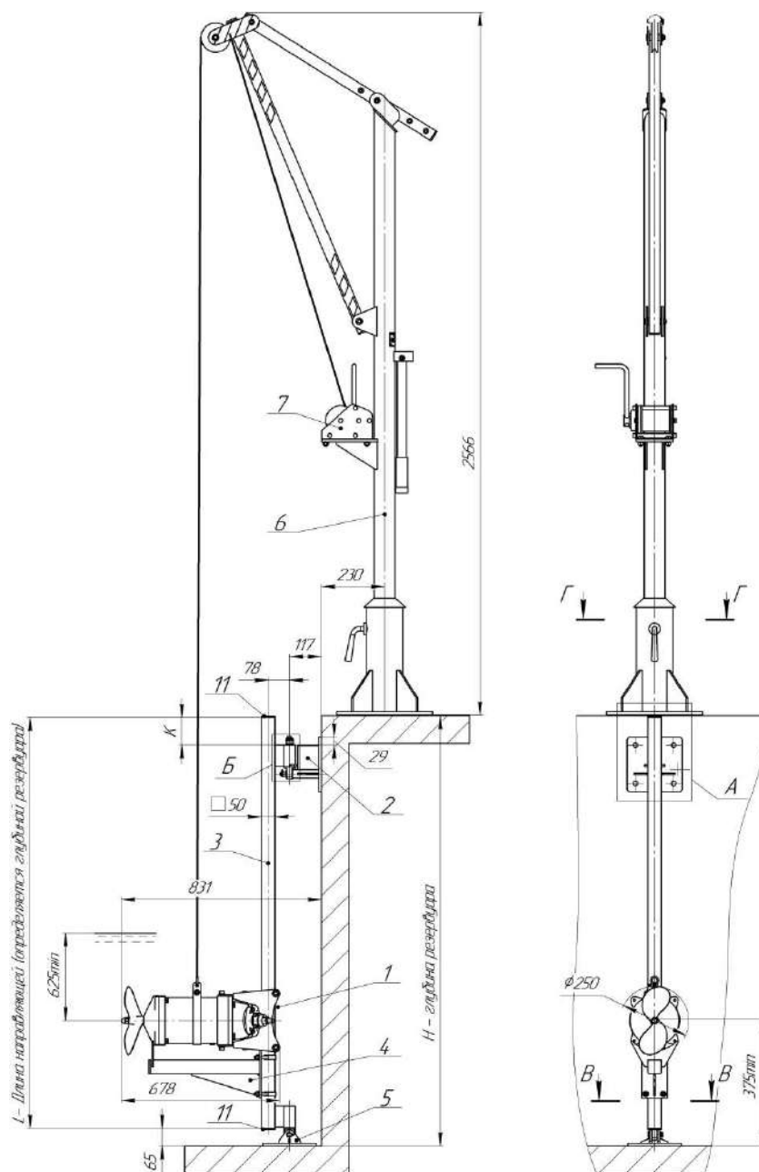
Рис. 1 Общий вид и габариты мешалки "Иртыш" Иртыш ПМ2 250-1,5/8-116
