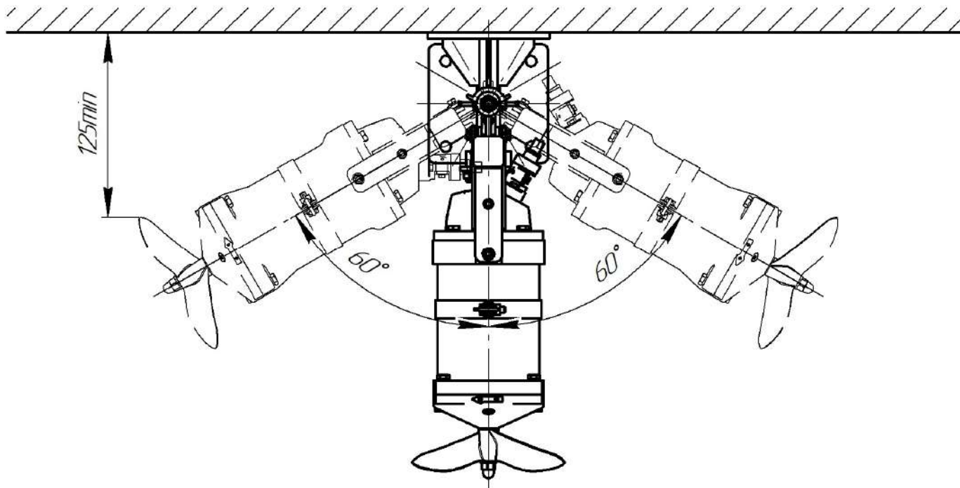
Рис. 2 Углы установки мешалки "Иртыш" ПМ2 250-1,5/8-116 в горизонтальной плоскости.
