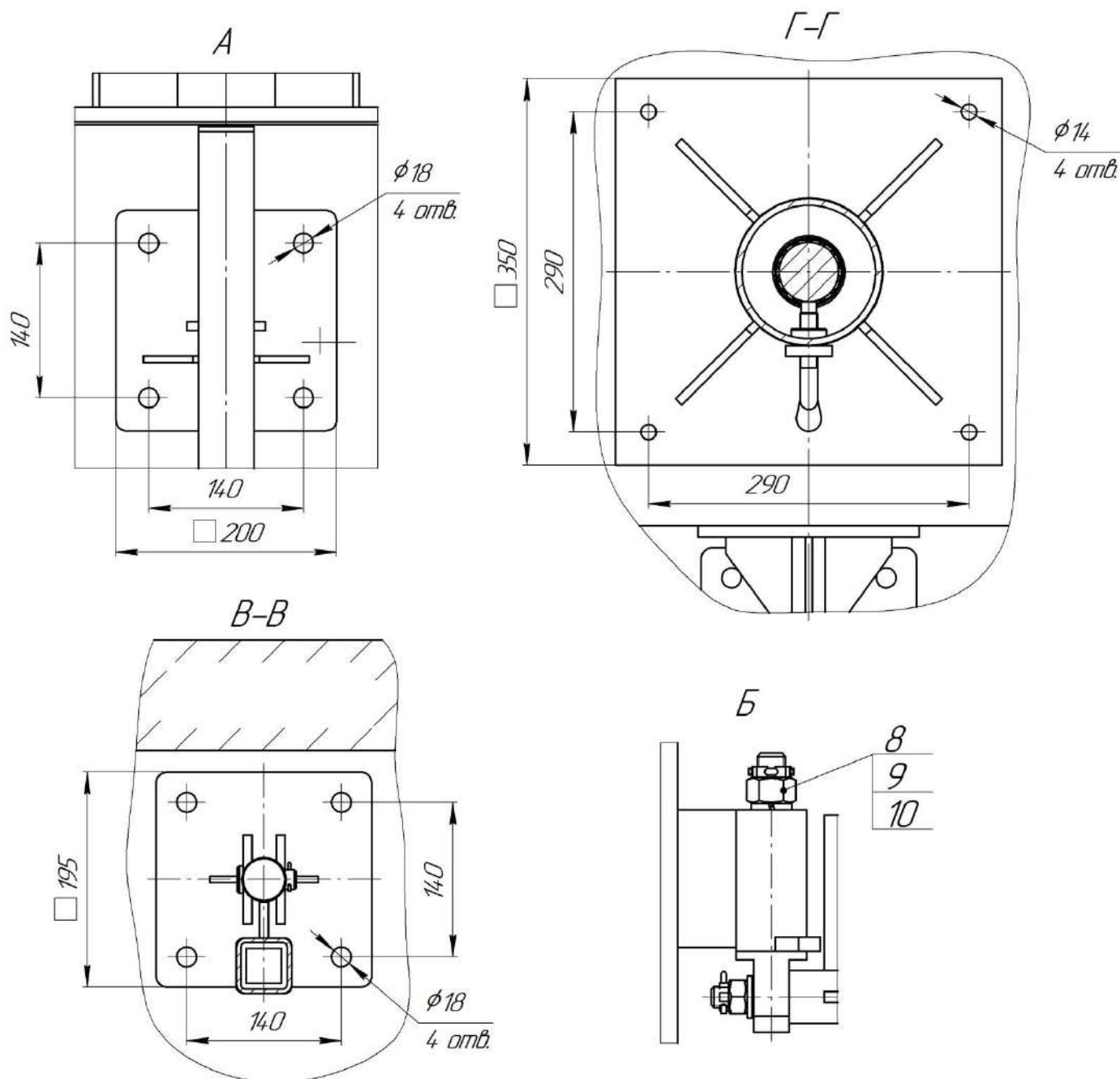
Рис. 1. Общий вид и габариты мешалки "Иртыш" Иртыш ПМ2 250-1,5/8-116 с опускным устройством и грузоподъемным механизмом.
