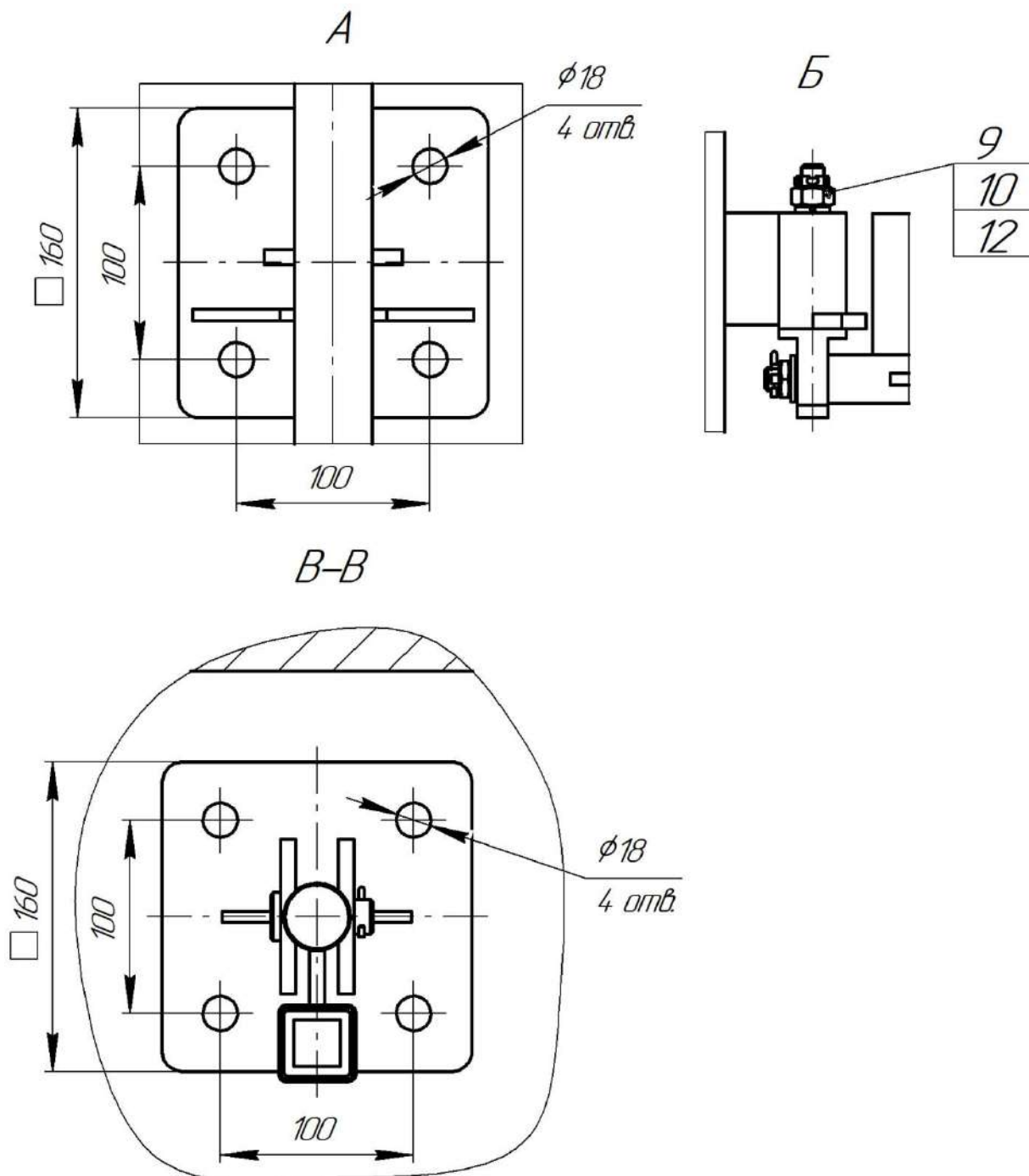
Рис. 1. Общий вид и габариты мешалки "Иртыш" ПМ2 250-2,2/6-116 с опускаемым устройством и грузоподъемным механизмом.
