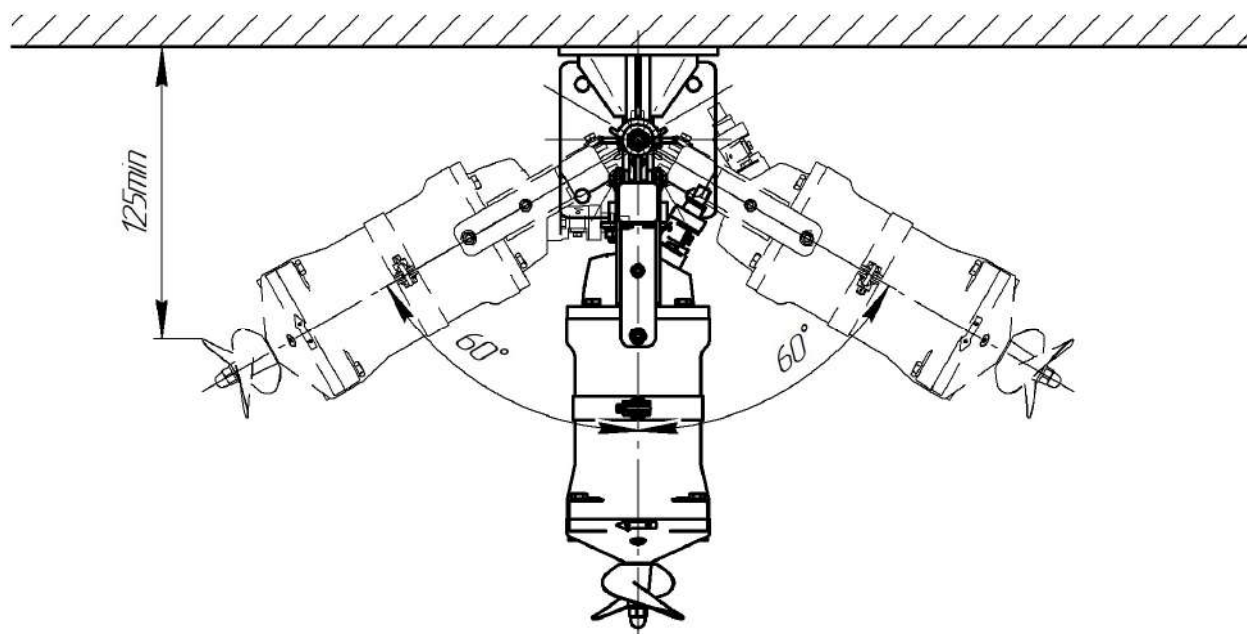
Рис. 2 Углы установки мешалка "Иртыш" ПМ2 250-2,2/6-116 в горизонтальной плоскости.
