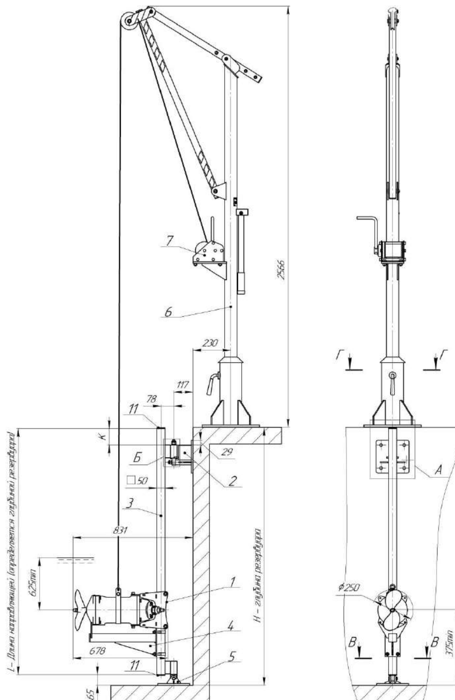
Рис. 1 Общий вид и габариты мешалки "Иртыш" ПМ2 250-2,2/6-116
