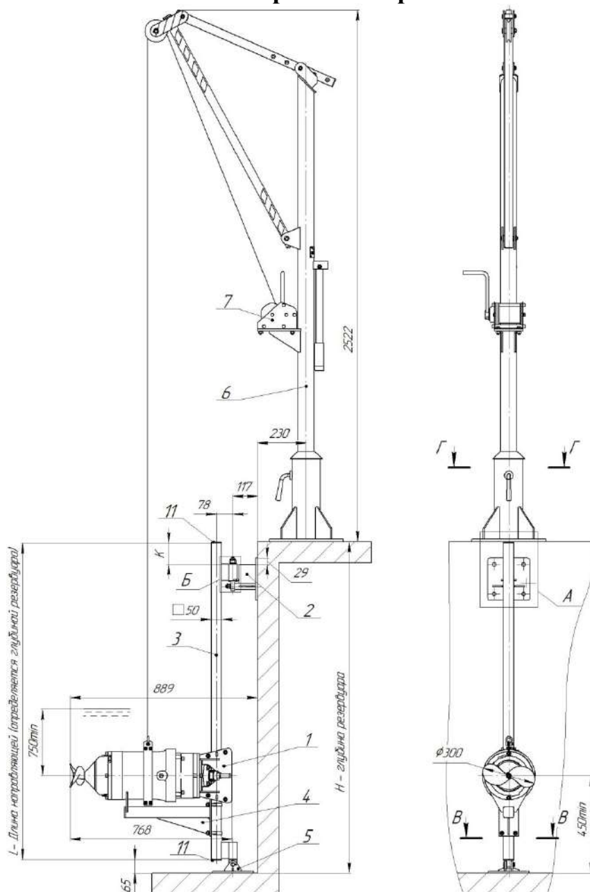
Рис. 1 Общий вид и габариты мешалки "Иртыш" Иртыш ПМ2 300-4/6-116
