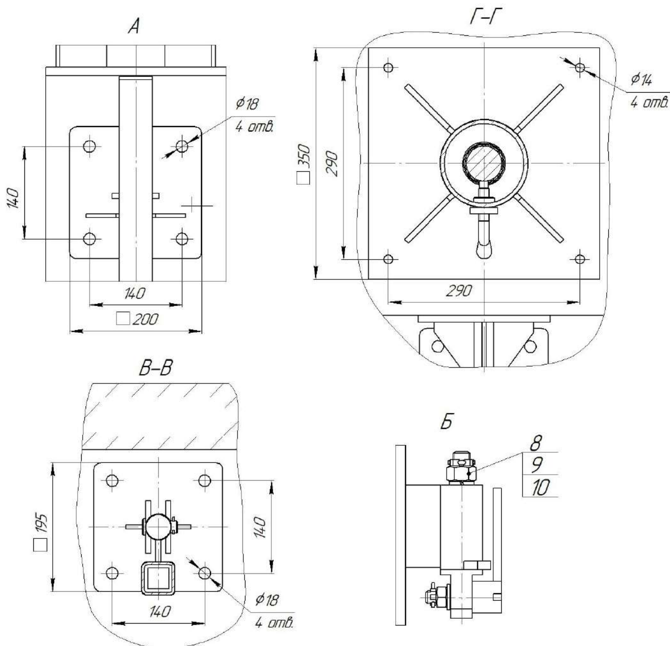
Рис. 1. Общий вид и габариты мешалки "Иртыш" Иртыш ПМ2 300-4/6-116 с опускным устройством и грузоподъемным механизмом.
