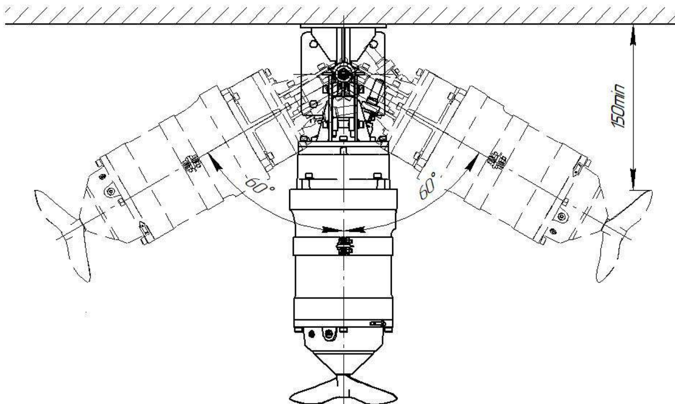
Рис. 2 Углы установки мешалки "Иртыш" ПМ2 300-4/6-116 в горизонтальной плоскости.
