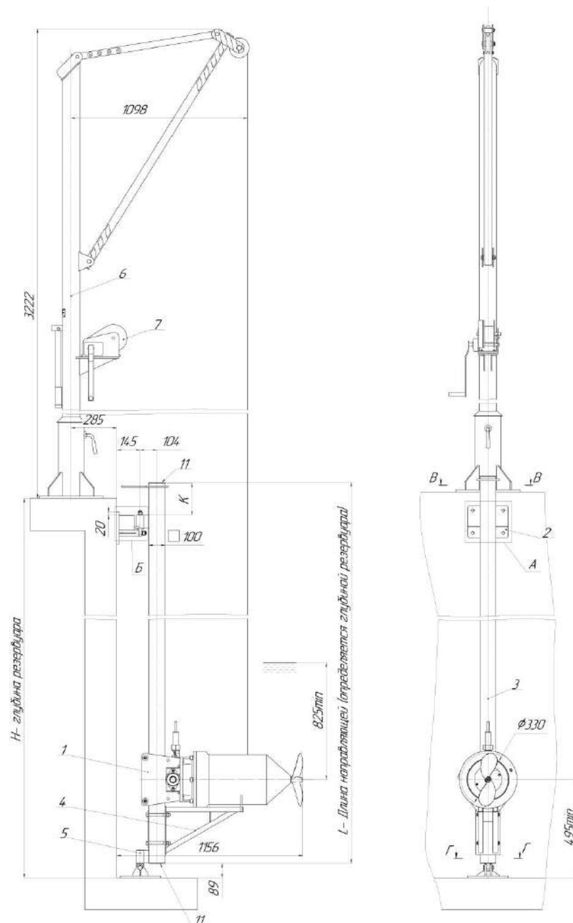
Рис. 1 Общий вид и габариты мешалки "Иртыш" ПМ2 330-18,5/4-116
