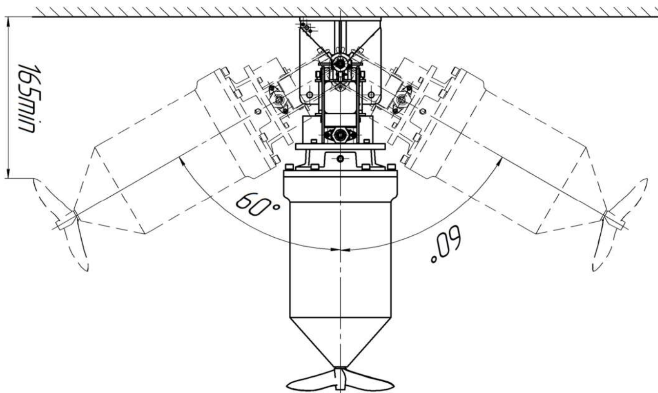
Рис. 2 Углы установки мешалки "Иртыш" ПМ2 330-18,5/4-116 в горизонтальной плоскости.
