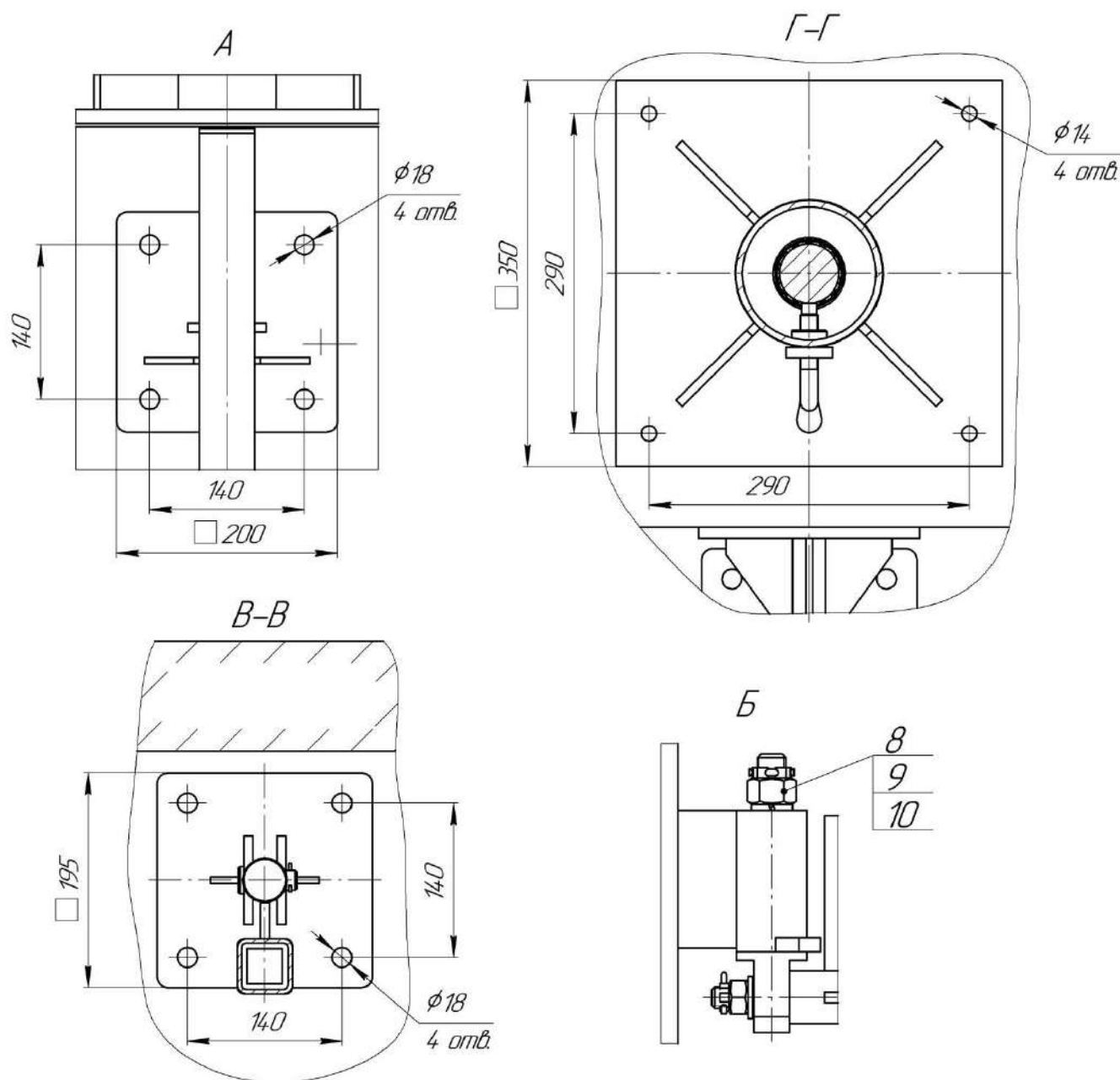
Рис. 1 Общий вид и габариты мешалки "Иртыш" ПМ2 330-5,5/6-116 с опускающим устройством и грузоподъёмным механизмом.
