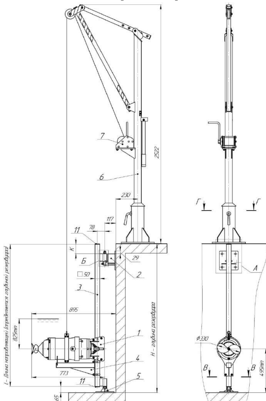
Рис. 1 Общий вид и габариты мешалки "Иртыш" ПМ2 330-5,5/6-116
