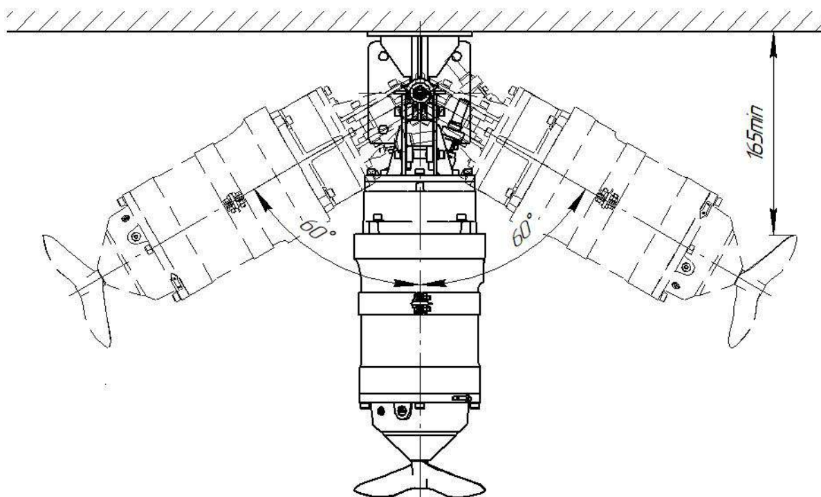
Рис. 2 Углы установки мешалки "Иртыш" ПМ2 330-5,5/6-116 в горизонтальной плоскости.
