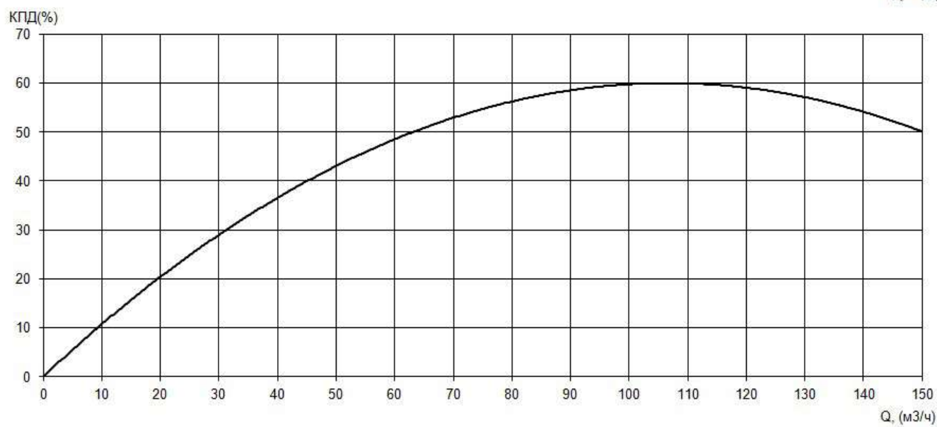
Рабочие характеристики насоса серии «Иртыш» НФ2 100/310.291-11/4
