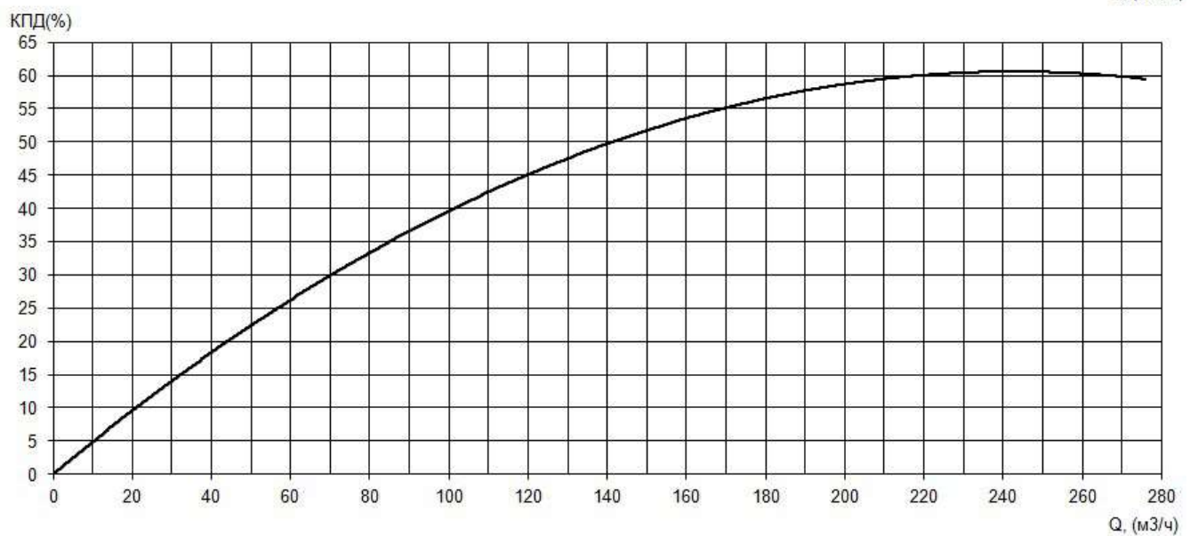
Рабочие характеристики насоса серии «Иртыш» НФ2 125/400.356-37/4
