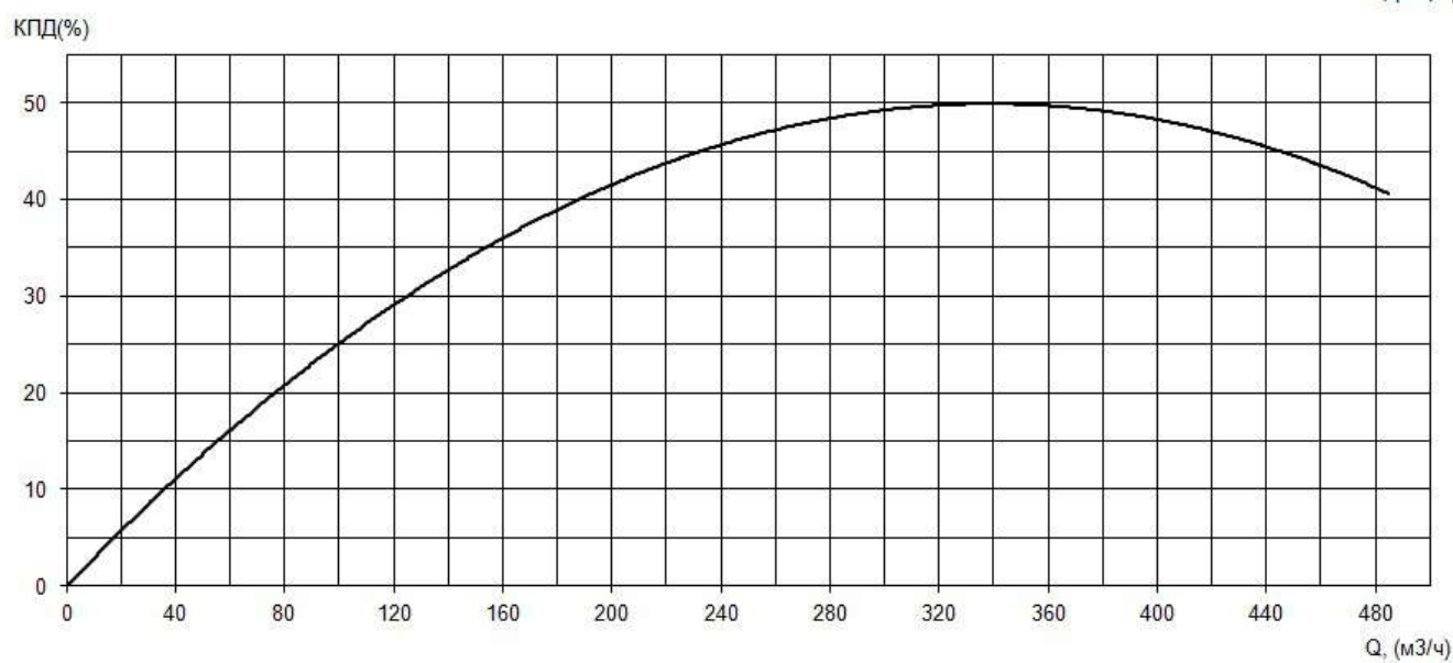
Рабочие характеристики насоса серии «Иртыш» НФ2 150/315.321-37/4
