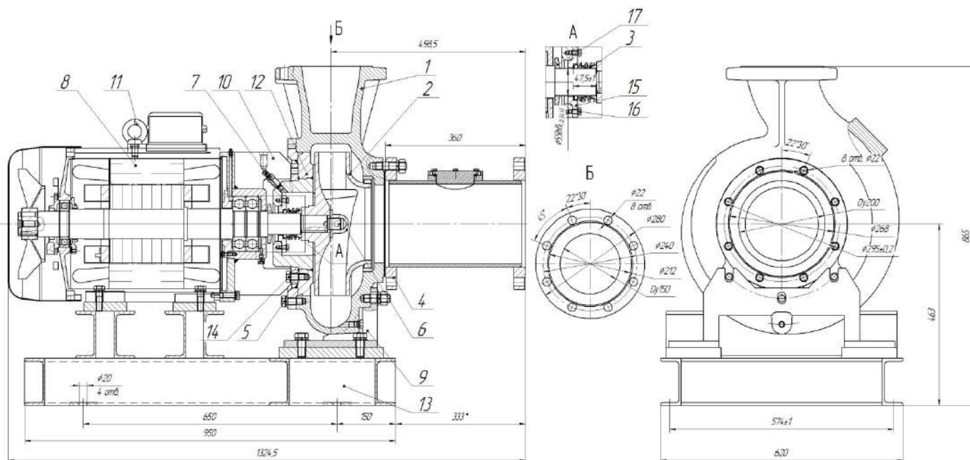
Общий вид и габаритные размеры электронасоса серии «Иртыш» НФ2 150/315.321-37/4-200
