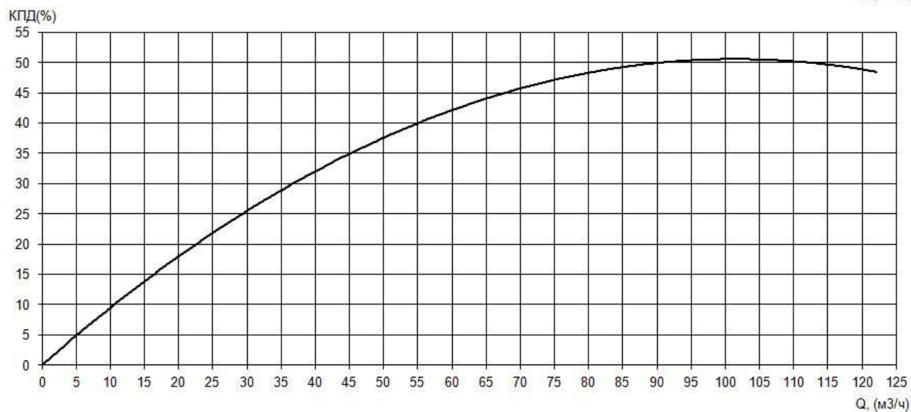
Рабочие характеристики насоса серии «Иртыш» НФ2 65/200.189-22/2
