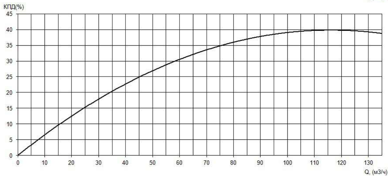
Рабочие характеристики насоса серии «Иртыш» НФс 100/310.301-18,5/4
