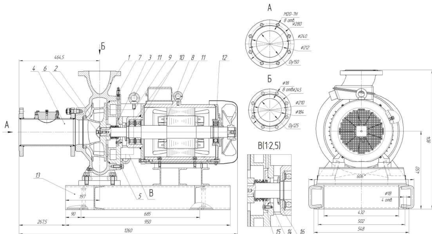
Общий вид и габаритные размеры электронасоса серии «Иртыш» НФ2 125/315.287-22/4-200
