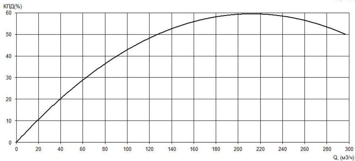
Рабочие характеристики насоса серии «Иртыш» НФ2 125/315.287-22/4
