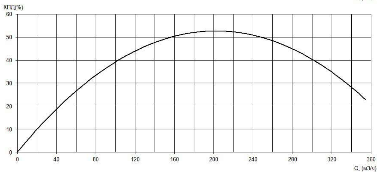
Рабочие характеристики насоса серии «Иртыш» НФ2 125/400.328-37/4
