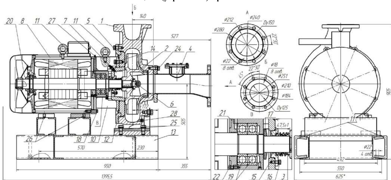
Общий вид, габаритные и присоединительные размеры электронасоса «Иртыш» НФ2 125/400.328-37/4-200
