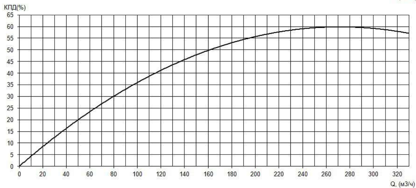
Рабочие характеристики насоса серии «Иртыш» НФ2 125/400.401-55/4
