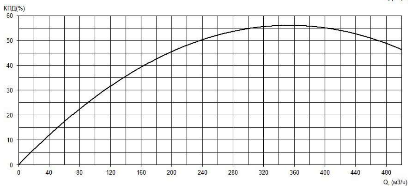
Рабочие характеристики насоса серии «Иртыш» НФ2 150/315.321-45/4
