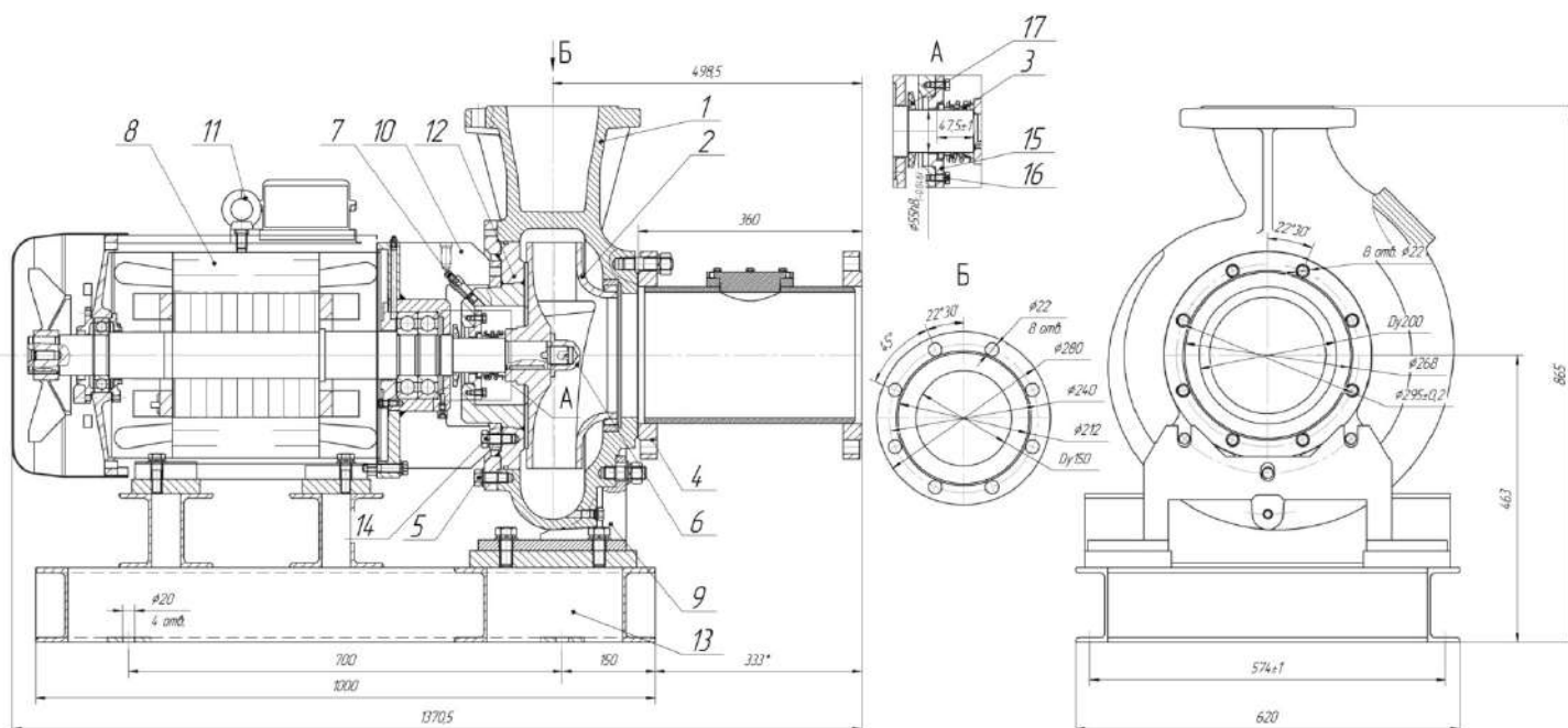
Общий вид и габаритные размеры электронасоса серии «Иртыш» НФ2 150/315.349-45/4-200
