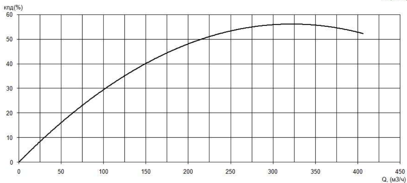
Рабочие характеристики насоса серии «Иртыш» НФ2 150/315.349-45/4
