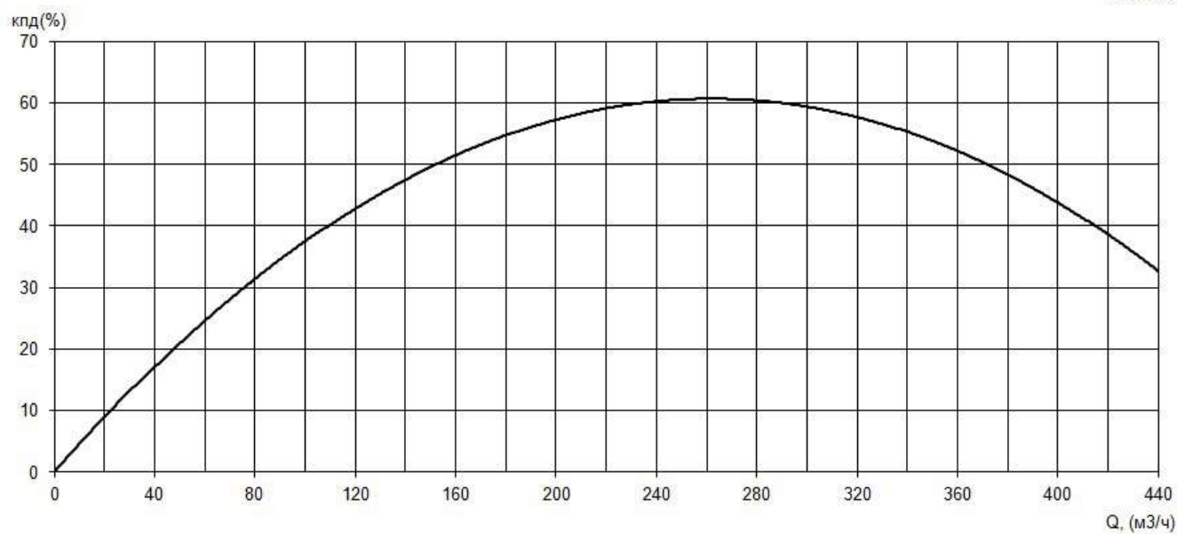
Рабочие характеристики насоса серии «Иртыш» НФ2 200/265.249-15/4
