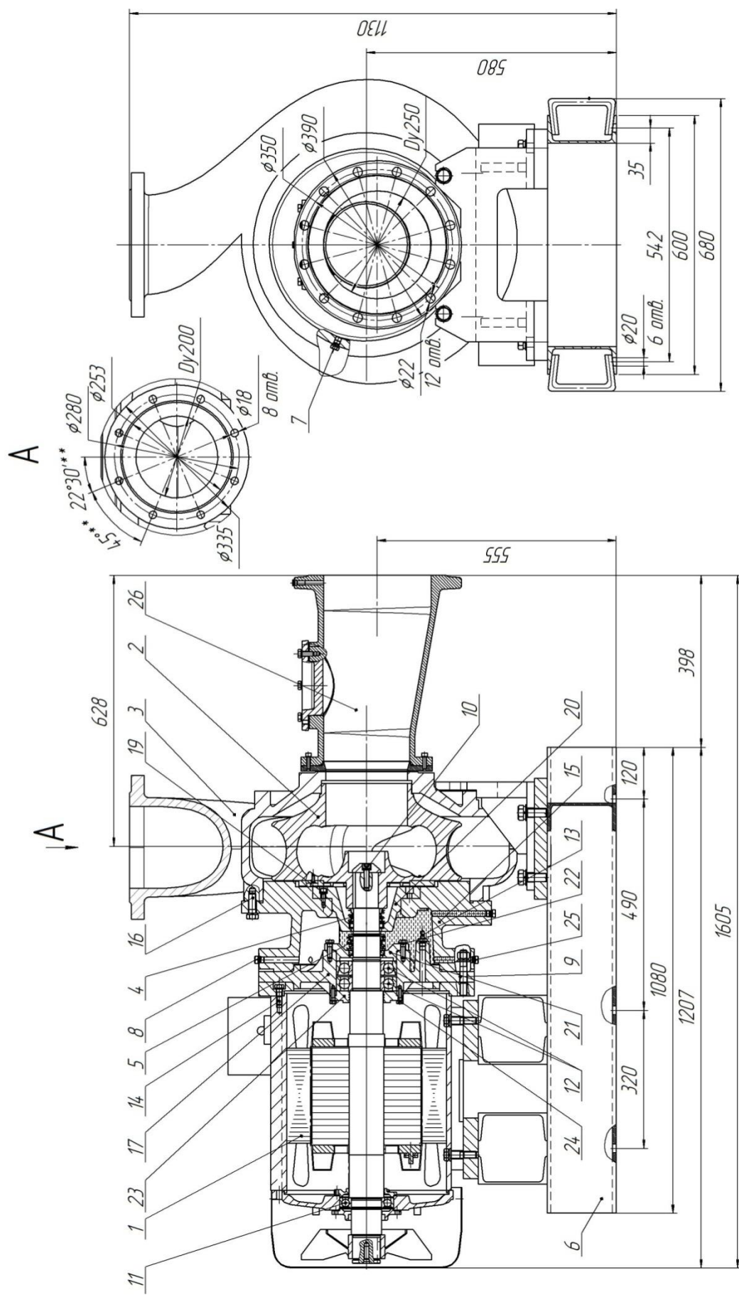
Приложение 1. Рис. 2. Общий вид, габаритные и присоединительные размеры электронасоса серии «Иртыш» НФ2 200/450.440-37/6-202.
