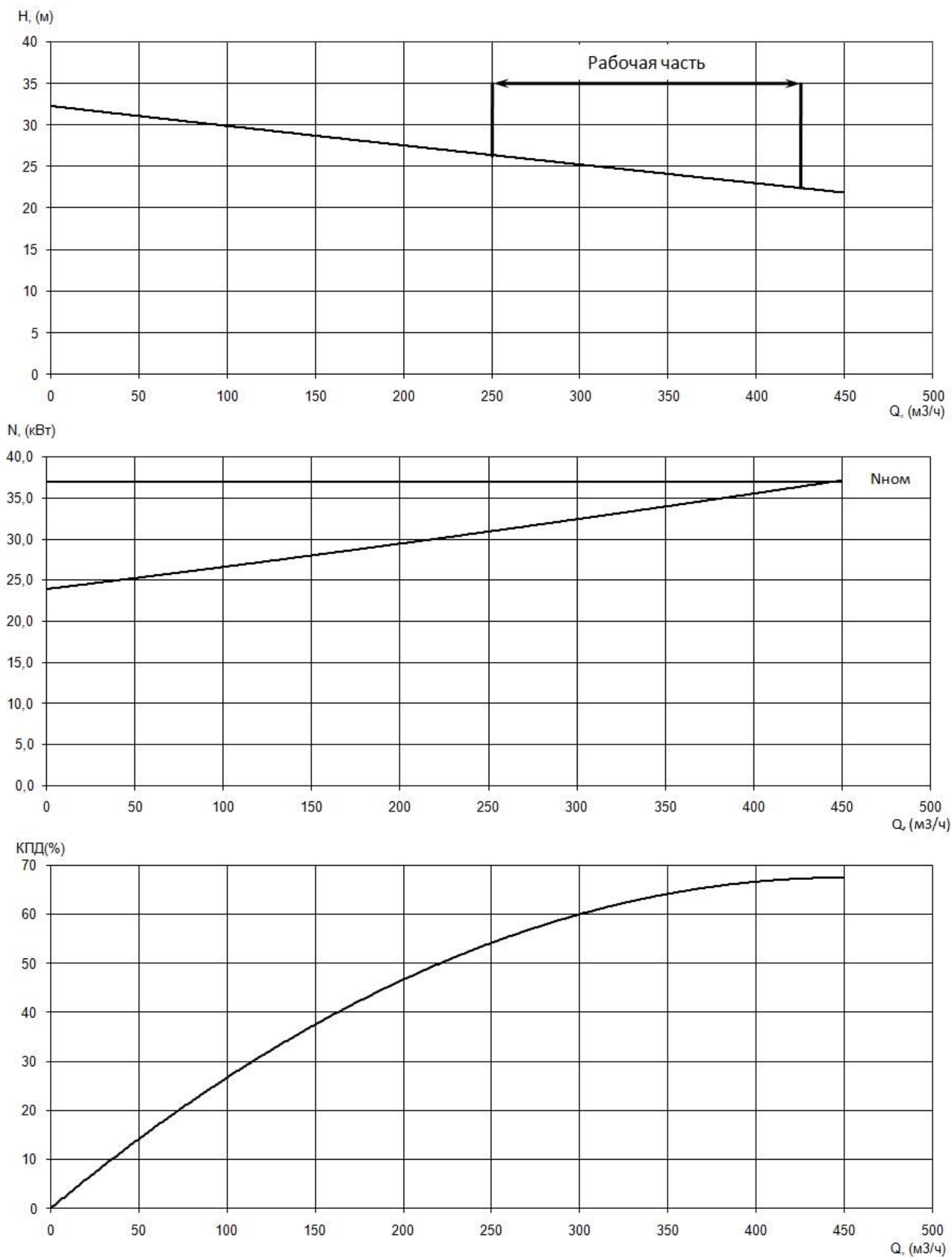
Приложение 1 Рис. 1. Рабочие характеристики электронасоса серии «Иртыш» НФ2 200/450.440-37/6.
