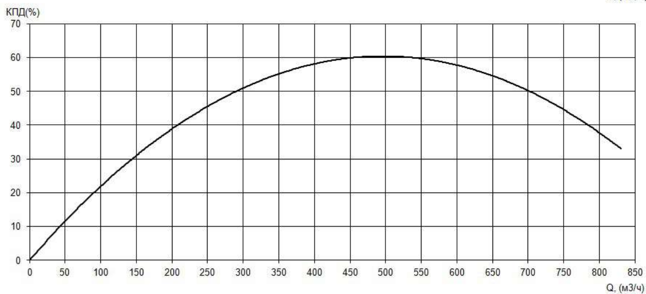
Рабочие характеристики насоса серии «Иртыш» НФ2 250/400.394-37/6
