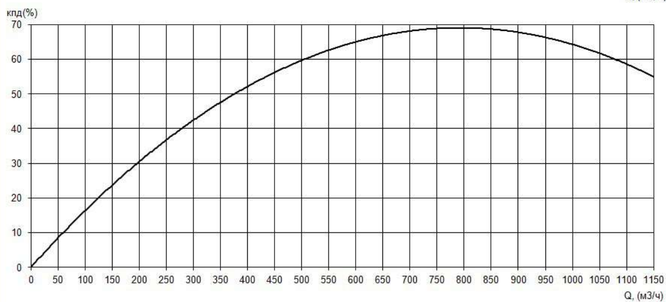
Рабочие характеристики насоса серии «Иртыш» НФ2 250/500.544-110/6
