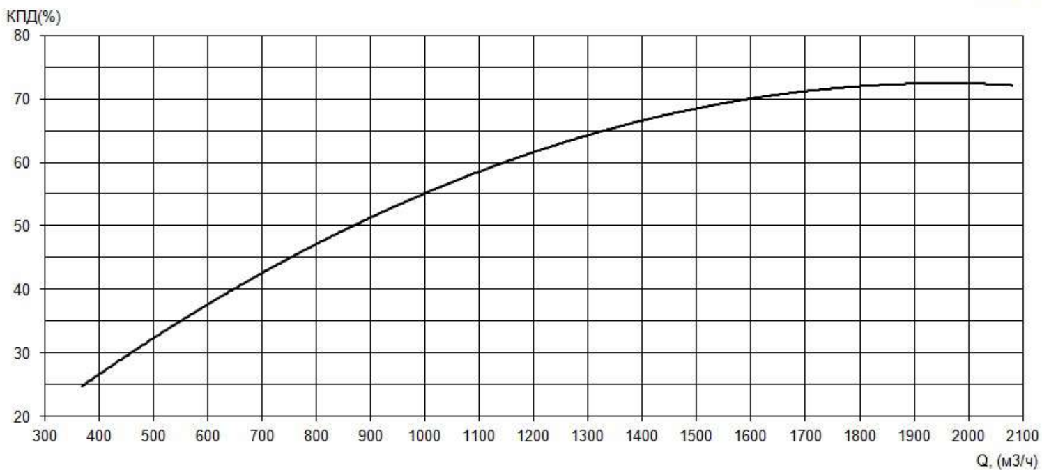
Рабочие характеристики насоса серии «Иртыш» НФ2 400/750.740-250/8
