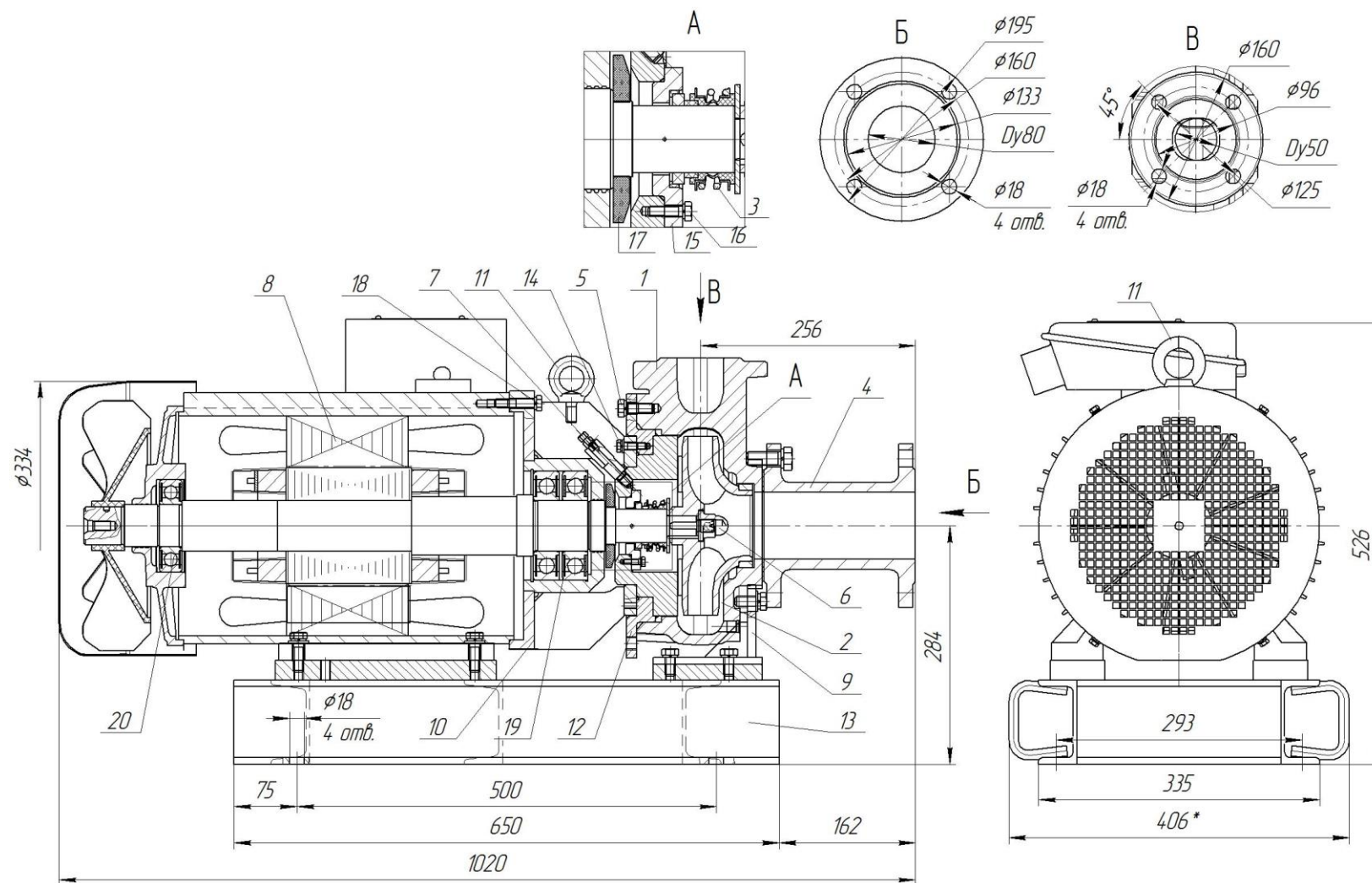
Приложение 1 Рис.2 Общий вид, габаритные и присоединительные размеры электронасоса серии «Иртыш» НФ2 50/200.212-18,5/2-200.
