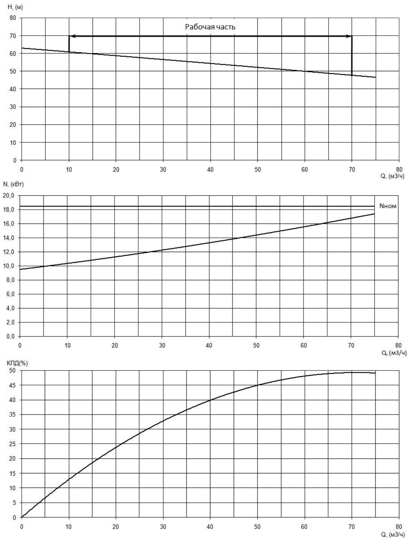
Приложение 1 Рис. 1. Рабочие характеристики электронасоса серии «Иртыш» НФ2 50/200.212-18,5/2.
