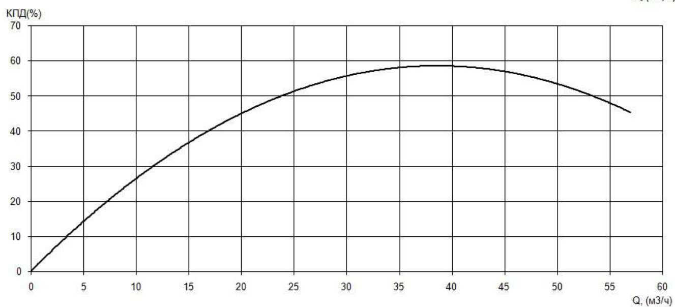
Рабочие характеристики насоса серии «Иртыш» НФ2 65/135.123-3/2
